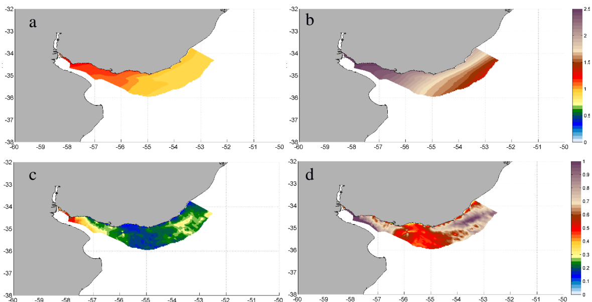
Figura 2. Mapas espaciales de (a,b) nivel del mar (m) y (c,d) intensidad de la corriente (m/s) en la franja costera y plataforma continental de Uruguay. La columna izquierda corresponde a los valores medios anuales mientras que la de la derecha, al percentil del 99% para el periodo 1985-2016.
