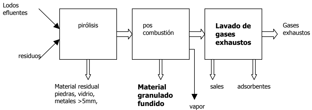
Proceso Schwel-Brenn
