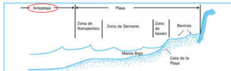
Figura 24. Esquema característico del perfil de una playa (requente).
