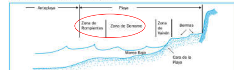
Figura 24. Esquema característico del perfil de una playa (resuelta).
