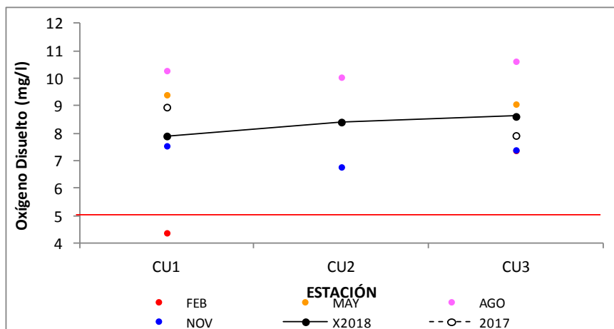
Figura 124. Variación del oxígeno disuelto en el agua, por estación de monitoreo, promedios 2017 y 2018.
