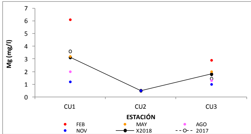
Figura 130. Variación del magnesio del agua, por estación de monitoreo, promedios 2017 y 2018.
