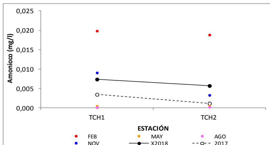
Figura 106. Variación de amoníaco, por estación de monitoreo, promedios 2017 y 2018.
