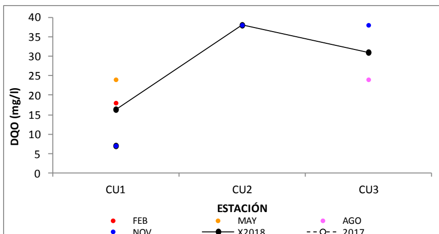
Figura 150. Variación de la DQO del agua, por estación de monitoreo, promedios 2017 y 2018.
