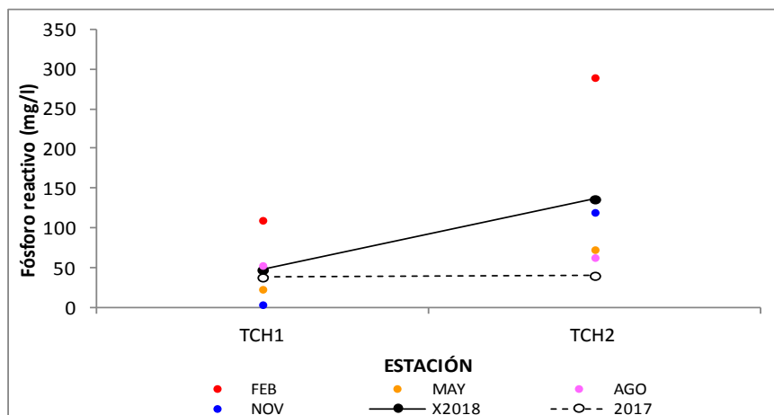
Figura 100. Variación del fósforo reactivo soluble, pro estación de monitoreo, promedios 2017 y 2018.
