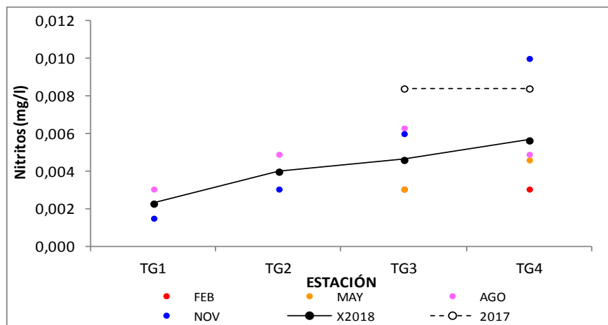
Figura 53. Variación de la concentración de nitrito, por estación de monitoreo, promedios 2017 y 2018.
