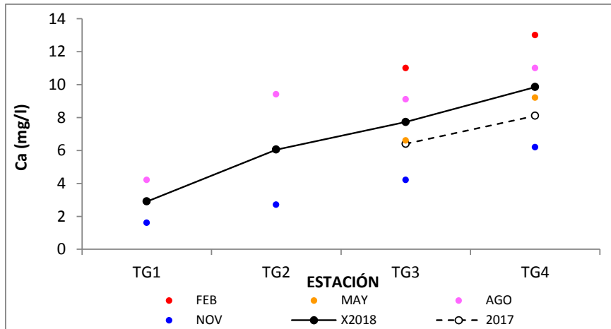
Figura 19. Variación de la concentración de calcio, por estación de monitoreo, promedios 2017 y 2018.
