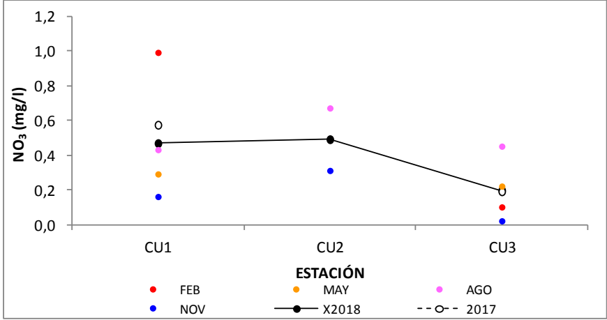
Figura 164. Variación del nitrato del agua, por estación de monitoreo, promedios 2017 y 2018.
