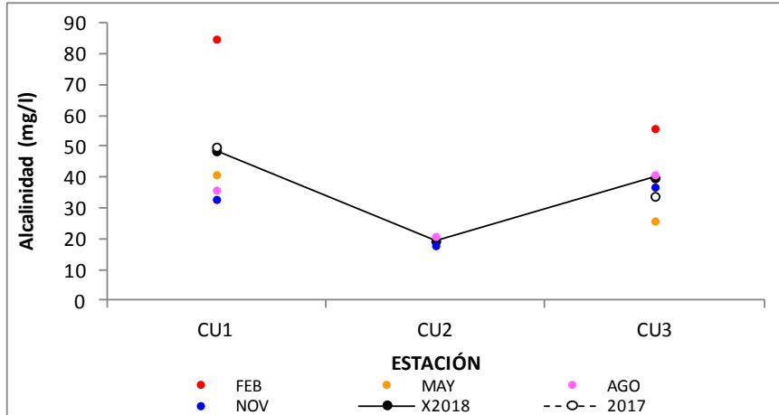
Figura 136. Variación de la alcalinidad total del agua, por estación de monitoreo, promedios 2017 y 2018.
