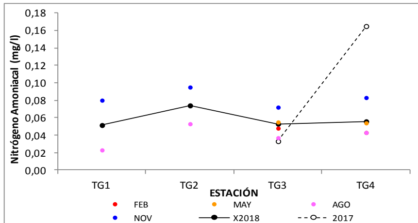
Figura 49. Izquierda: variación de la concentración de nitrógeno amoniacal, por estación de monitoreo, promedios 2017 y 2018.
