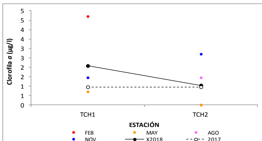
Figura 112. Variación de clorofila a , por estación de monitoreo, promedios 2017 y 2018.
