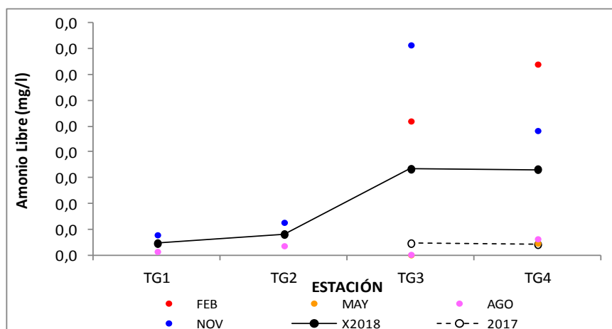
Figura 51. Variación de la concentración de amoniaco, por estación de monitoreo, promedios 2017 y 2018.
