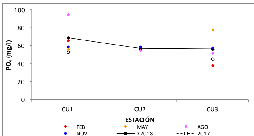
Figura 154. Variación del fósforo reactivo del agua, por estación de monitoreo, promedios 2017 y 2018.
