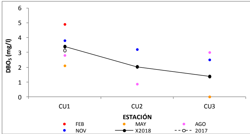
Figura 148. Variación de la DBO 5 del agua, por estación de monitoreo, promedios 2017 y 2018.
