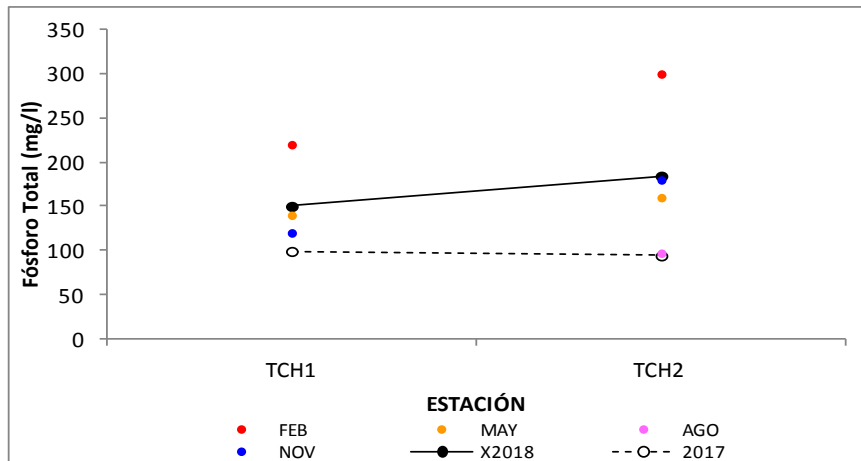
Figura 98. Variación del fósforo total, por estación de monitoreo, promedios 2017 y 2018.
