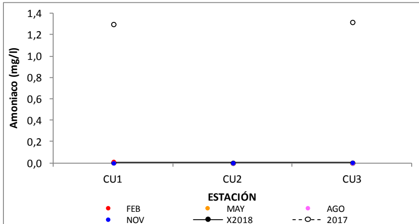
Figura 160. Variación del amoníaco del agua, por estación de monitoreo, promedios 2017 y 2018.
