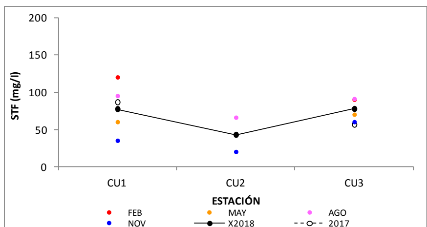
Figura 140. Variación de los sólidos totales fijos del agua, por estación de monitoreo, promedios 2017 y 2018.
