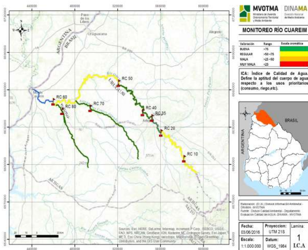
Figura 2.31 – Mapa de calidad de agua en base a la aplicación de índice de calidad
