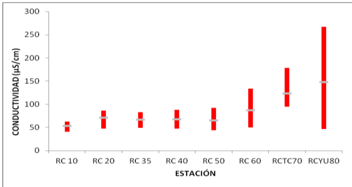
Figura 2.7 – Distribución espacial de la conductividad en el área de estudio. En gris: promedios anuales por estación, en rojo: máximos y mínimos por estación.
