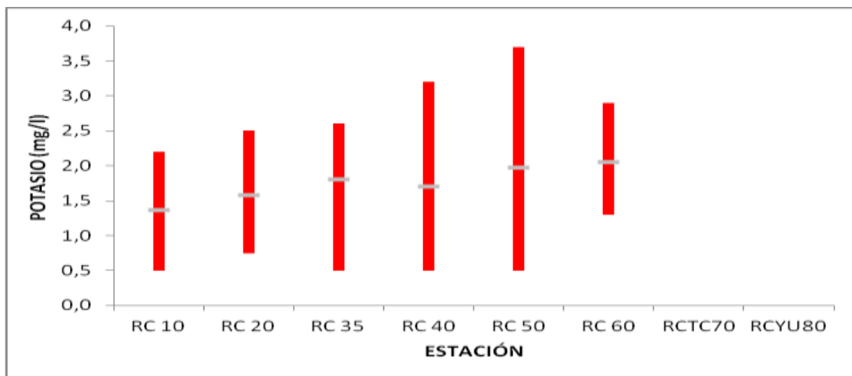
Figura 2.15 – Distribución espacial de potasio en el área de estudio. En gris: promedios anuales por estación, en rojo: máximos y mínimos por estación.
