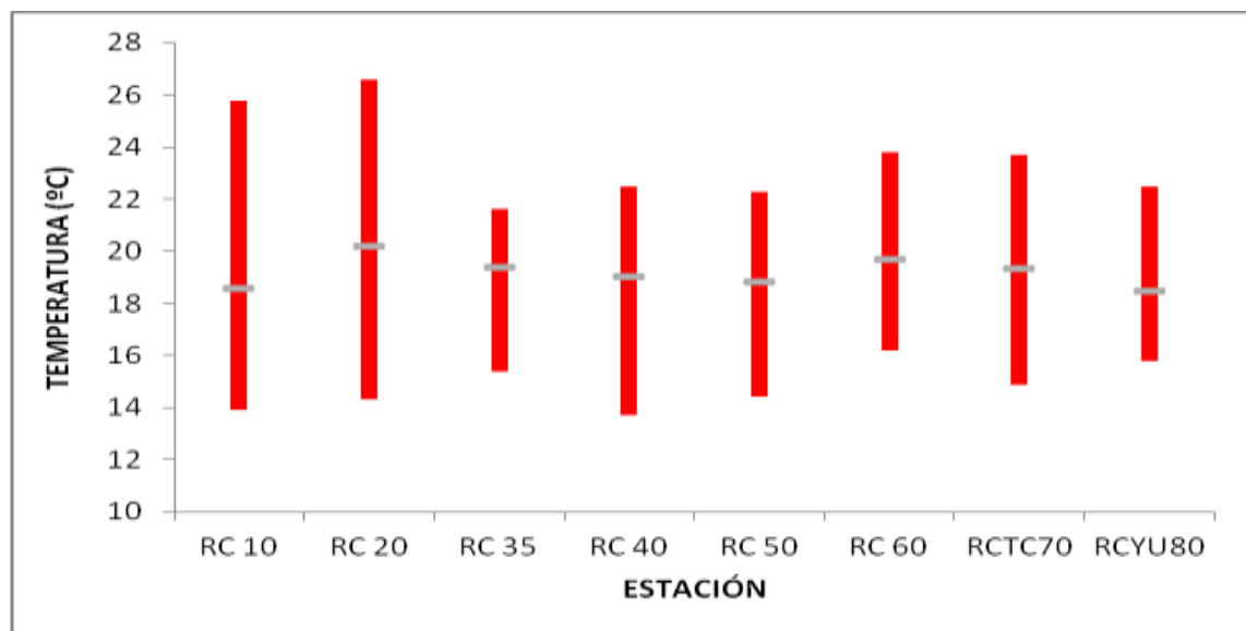
Figura 2.6 – Variación de la temperatura del agua entre los sitios de monitoreo. En gris: promedios anuales por estación, en rojo: máximos y mínimos por estación.
