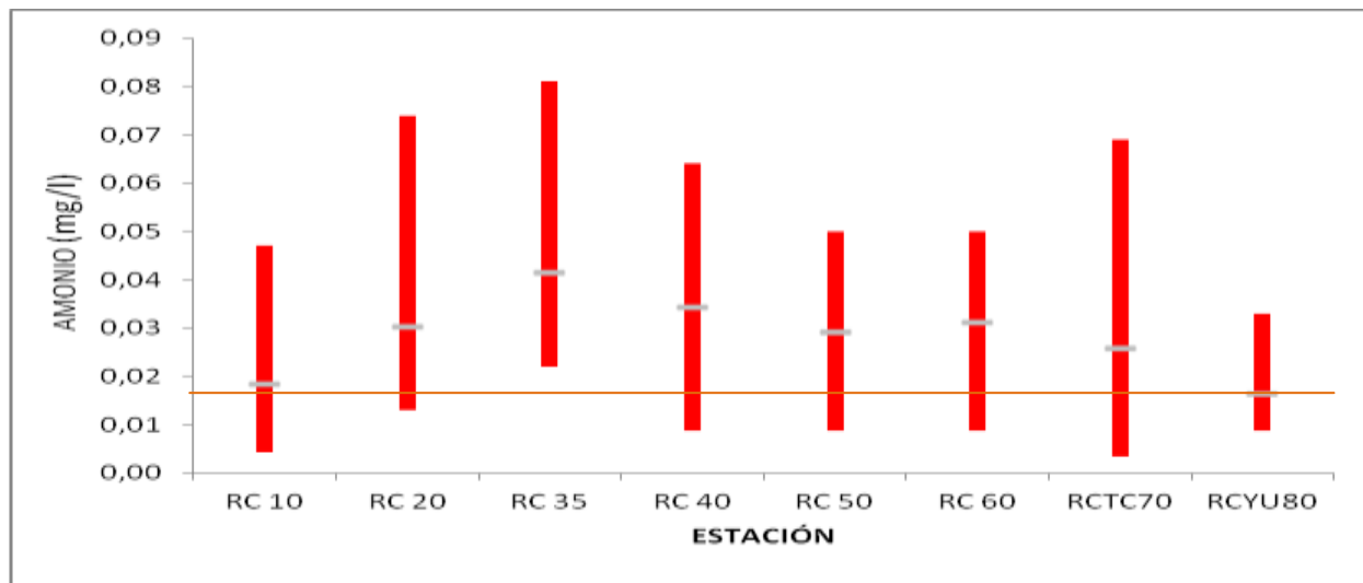
Figura 2.21 – Distribución espacial de amonio en el área de estudio. En gris: promedios anuales por estación, en rojo: máximos y mínimos por estación.
