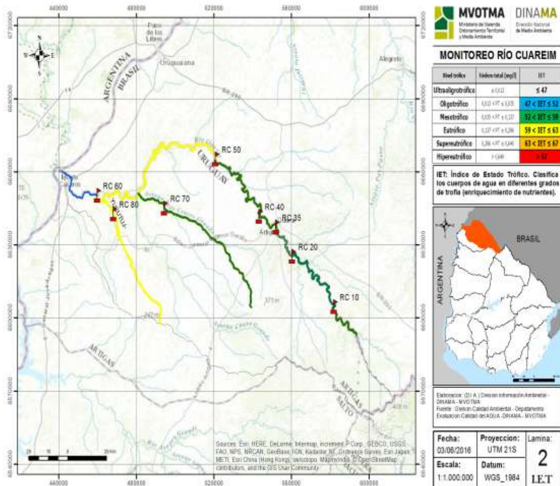
Figura 2.32 – Mapa de calidad de agua en base a la aplicación de índice de estado trófico
