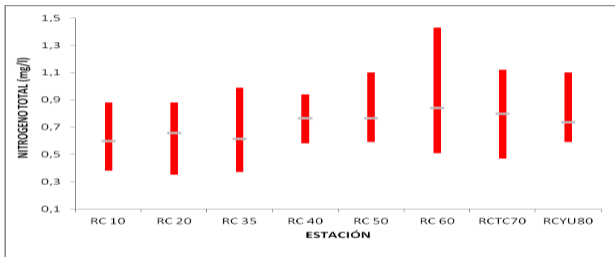
Figura 2.22 – Distribución espacial de nitrógeno total en el área de estudio En gris: promedios anuales por estación, en rojo: máximos y mínimos por estación.
