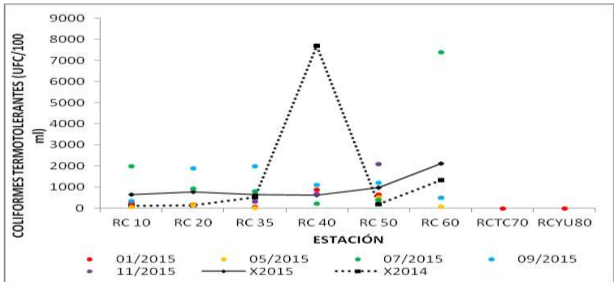
Figura 2.30 – Comparación de la distribución espacial de Coliformes Termotolerantes entre el periodo 2014 y el 2015
