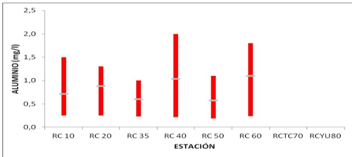
Figura 2.25 – Distribución espacial de aluminio en la zona de estudio. En gris: promedios anuales por estación, en rojo: máximos y mínimos por estación.
