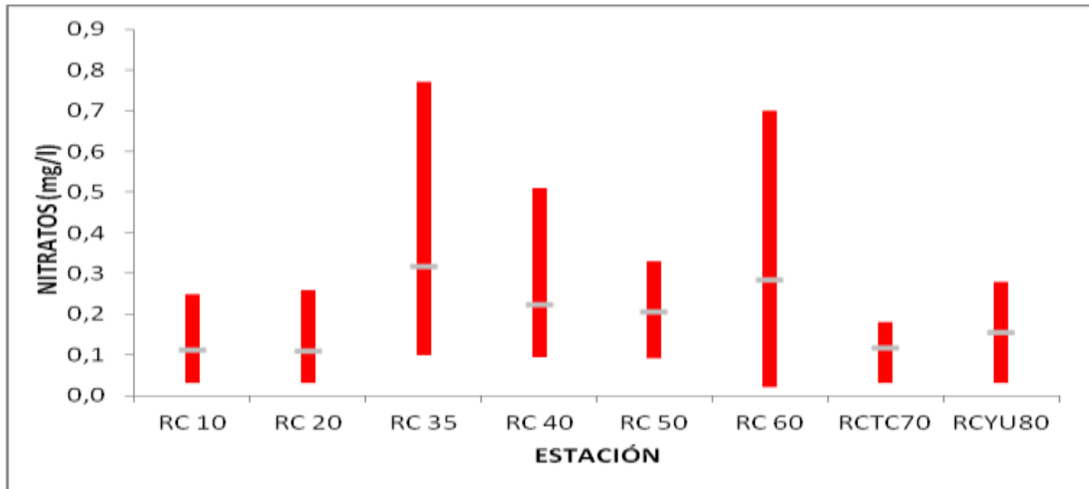
Figura 2.19 – Distribución espacial de nitratos en el área de estudio. En gris: promedios anuales por estación, en rojo: máximos y mínimos por estación.
