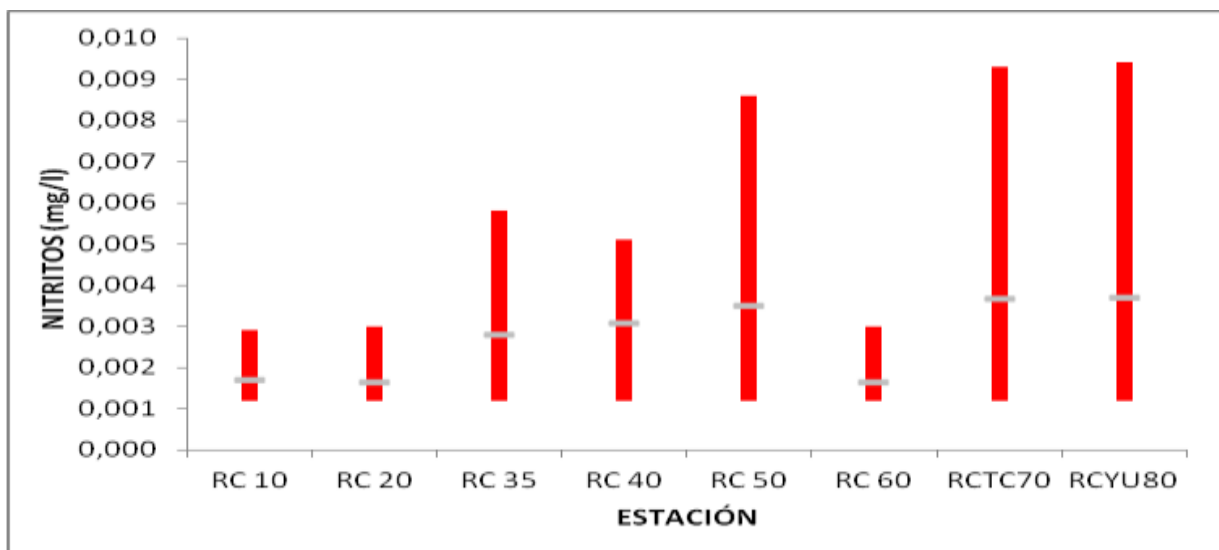
Figura 2.20 – Distribución espacial de nitritos en el área de estudio. En gris: promedios anuales por estación, en rojo: máximos y mínimos por estación.
