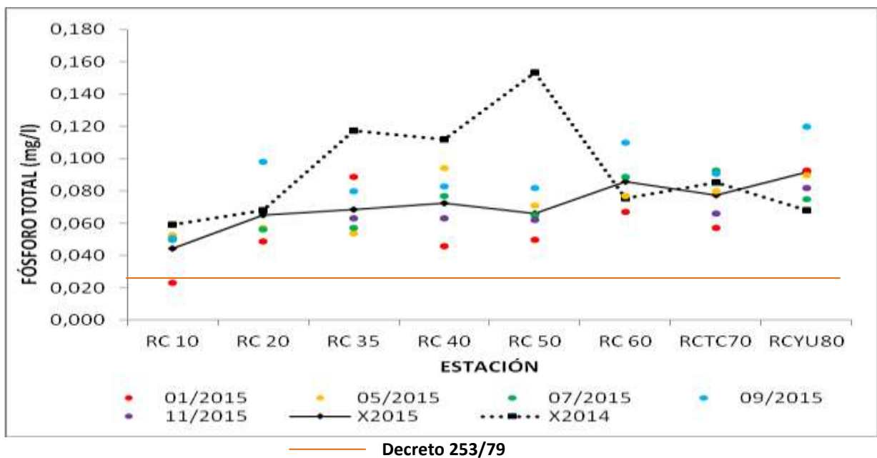
Figura 2.27 – Comparación de la distribución espacial de Fosforo Total entre el periodo 2014 y el 2015.
