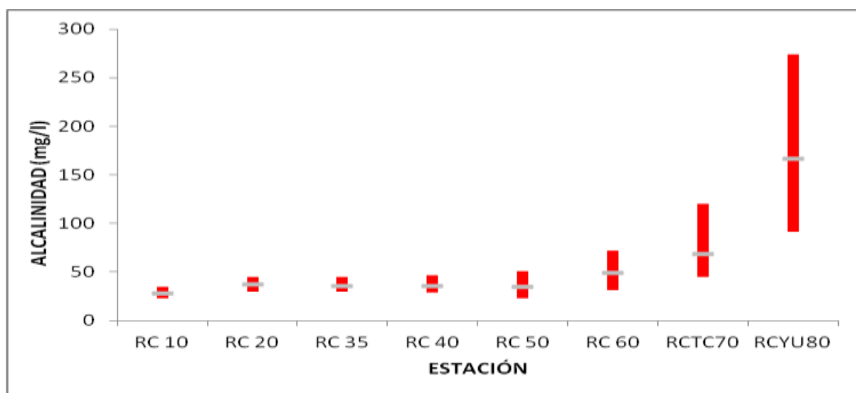
Figura 2.16 – Distribución espacial de alcalinidad en el área de estudio. En gris: promedios anuales por estación, en rojo: máximos y mínimos por estación.
