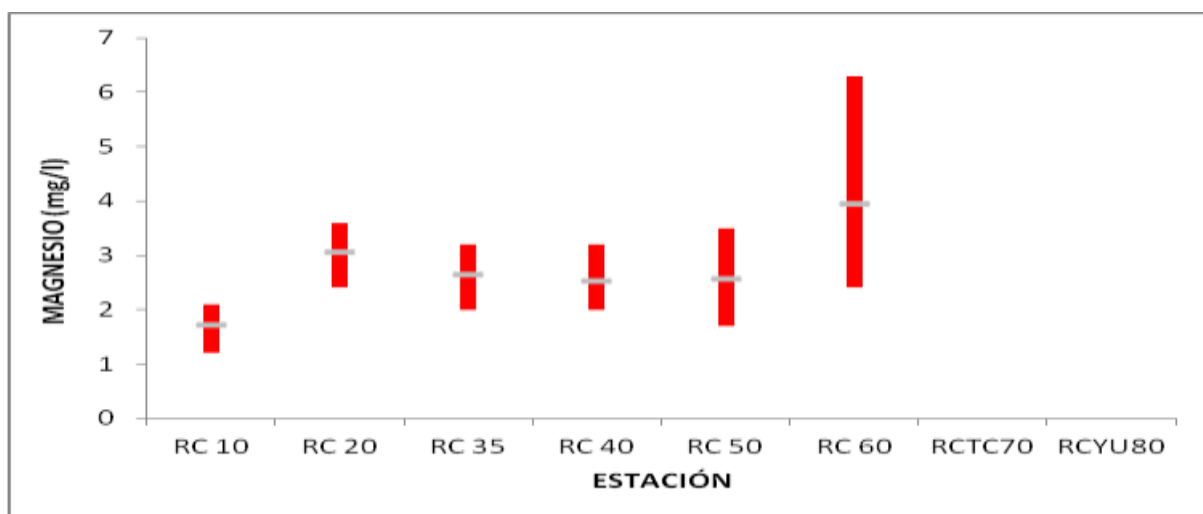
Figura 2.13 – Distribución espacial de magnesio en el área de estudio. En gris: promedios anuales por estación, en rojo: máximos y mínimos por estación.
