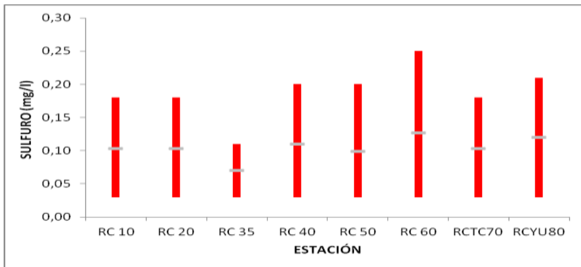
Figura 2.17 – Distribución espacial de sulfuros en el río Cuareim. En gris: promedios anuales por estación, en rojo: máximos y mínimos por estación.
