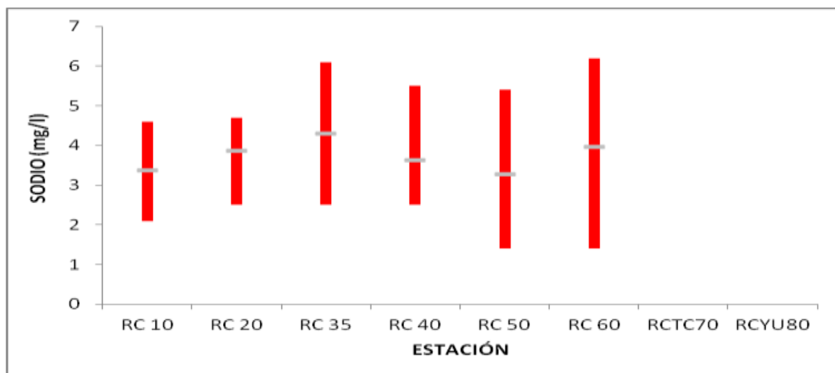
Figura 2.14 – Distribución espacial de sodio en el área de estudio. En gris: promedios anuales por estación, en rojo: máximos y mínimos por estación.
