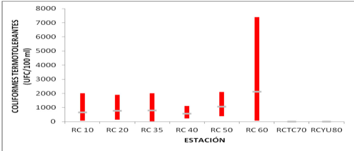
Figura 2.11 – Distribución espacial de Coliformes termotolerantes en el área de estudio. En gris: promedios anuales por estación, en rojo: máximos y mínimos por estación.
