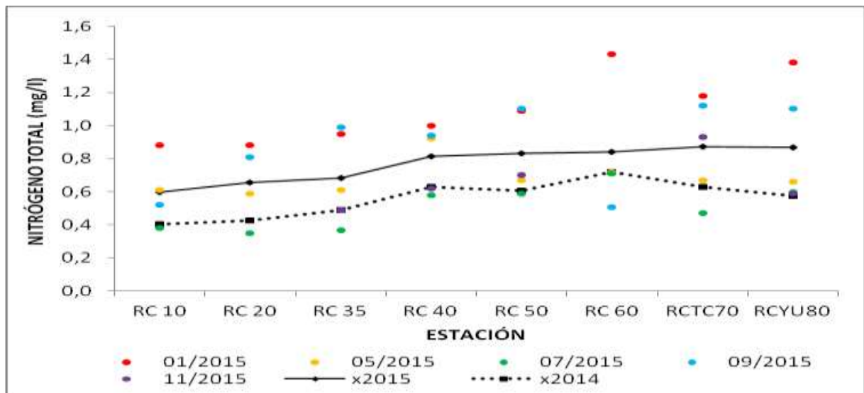
Figura 2.28 – Comparación de la distribución espacial de Nitrógeno Total entre el periodo 2014 y el 2015
