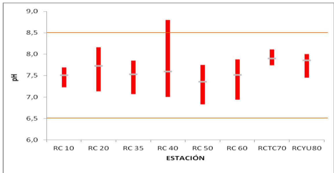
Figura 2.8 – Distribución espacial de pH por estación. En gris: promedios anuales por estación, en rojo: máximos y mínimos por estación.
