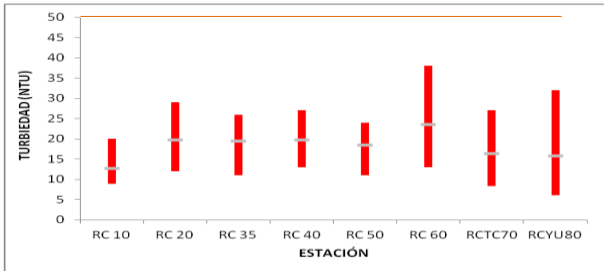
Figura 2.10 – Distribución espacial de turbiedad en el área de estudio En gris: promedios anuales por estación, en rojo: máximos y mínimos por estación.
