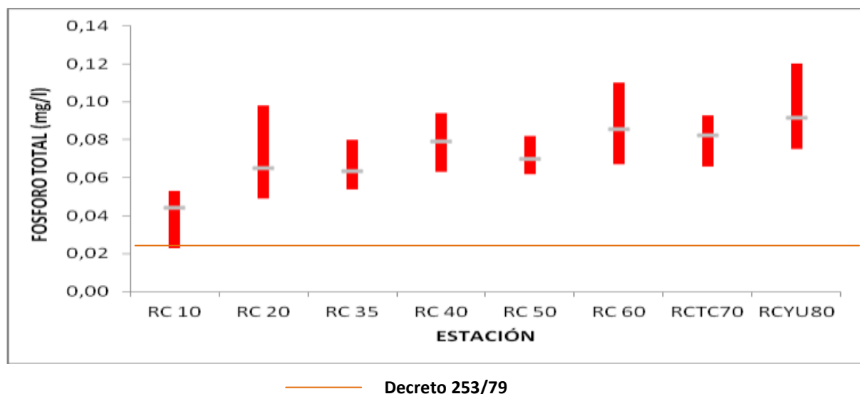
Figura 2.23 – Distribución espacial de fósforo total en el área de estudio. En gris: promedios anuales por estación, en rojo: máximos y mínimos por estación.
