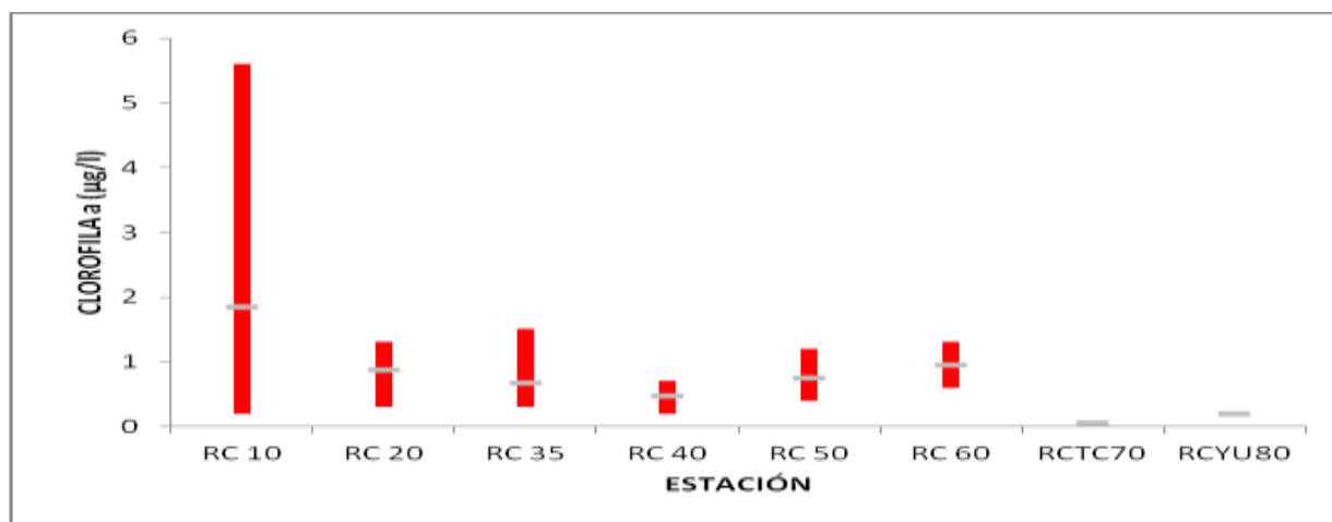
Figura 2.24 – Distribución espacial de la biomasa algal (clorofila-a) en el río Cuareim. En gris: promedios anuales por estación, en rojo: máximos y mínimos por estación.
