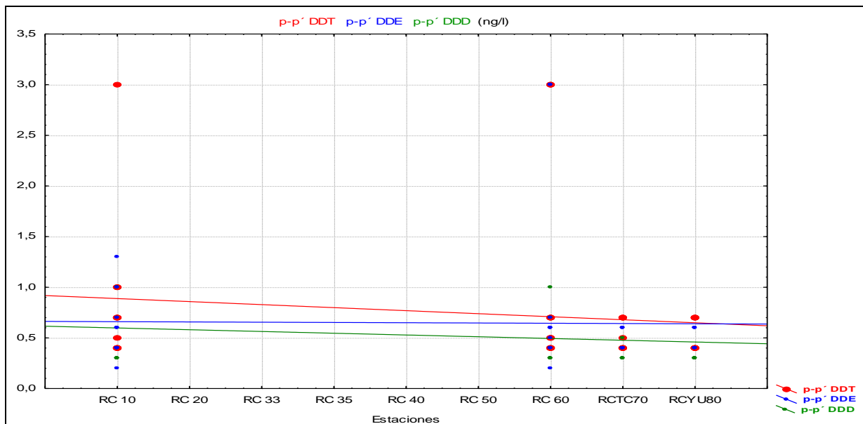
Figura 2.26 – Distribución espacial de DDE, DDD y DDT en las estaciones monitoreadas.
