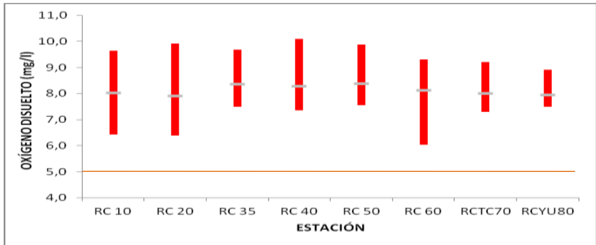
Figura 2.9 – Distribución espacial de oxígeno disuelto en el área de estudio En gris: promedios anuales por estación, en rojo: máximos y mínimos por estación.
