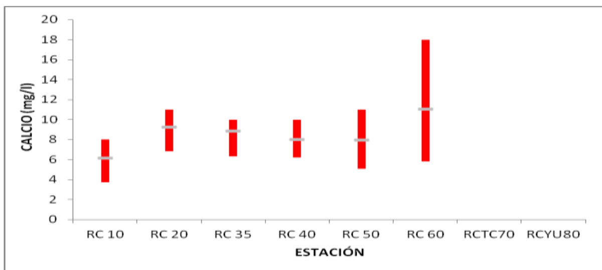
Figura 2.12 – Distribución espacial de calcio en el área de estudio. En gris: promedios anuales por estación, en rojo: máximos y mínimos por estación.
