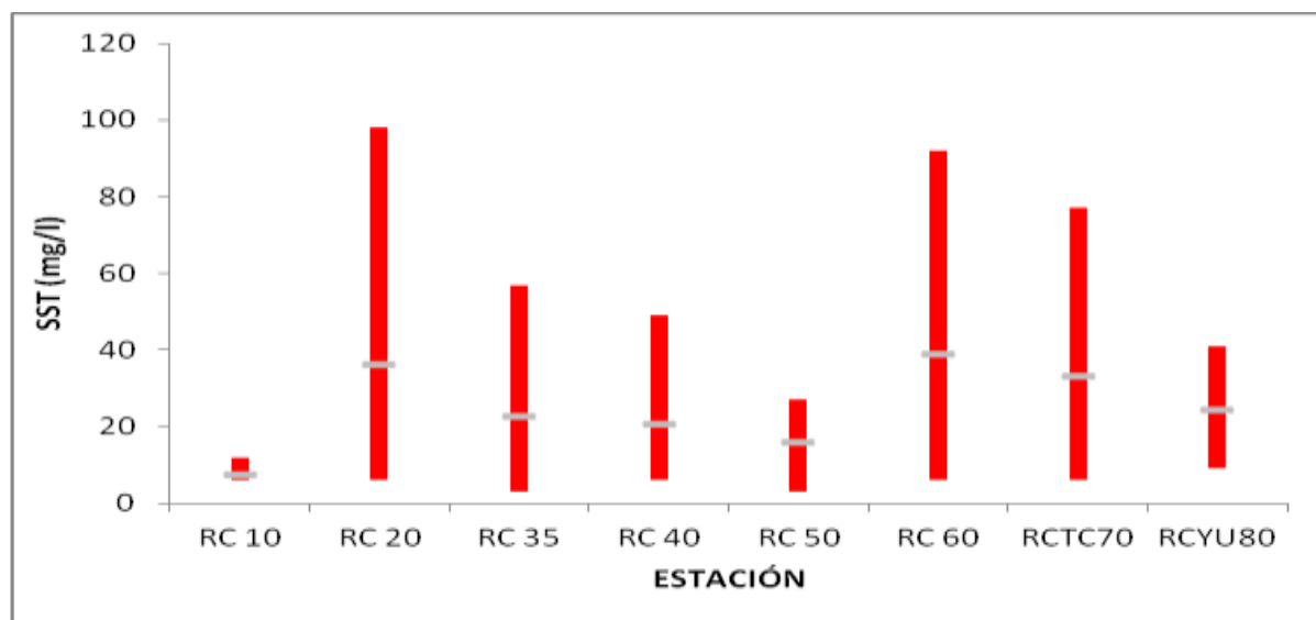
Figura 2.18 – Distribución espacial de sólidos suspendidos totales en el área de estudio. En gris: promedios anuales por estación, en rojo: máximos y mínimos por estación.
