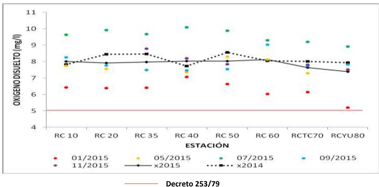
Figura 2.29 – Comparación de la distribución espacial de Oxígeno Disuelto entre el periodo 2014 y el 2015.
