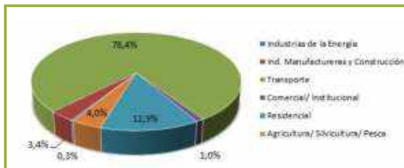
Figura 23: Participación de los sectores de actividad de quema de combustibles en las emisiones de COVDM, 2010.
