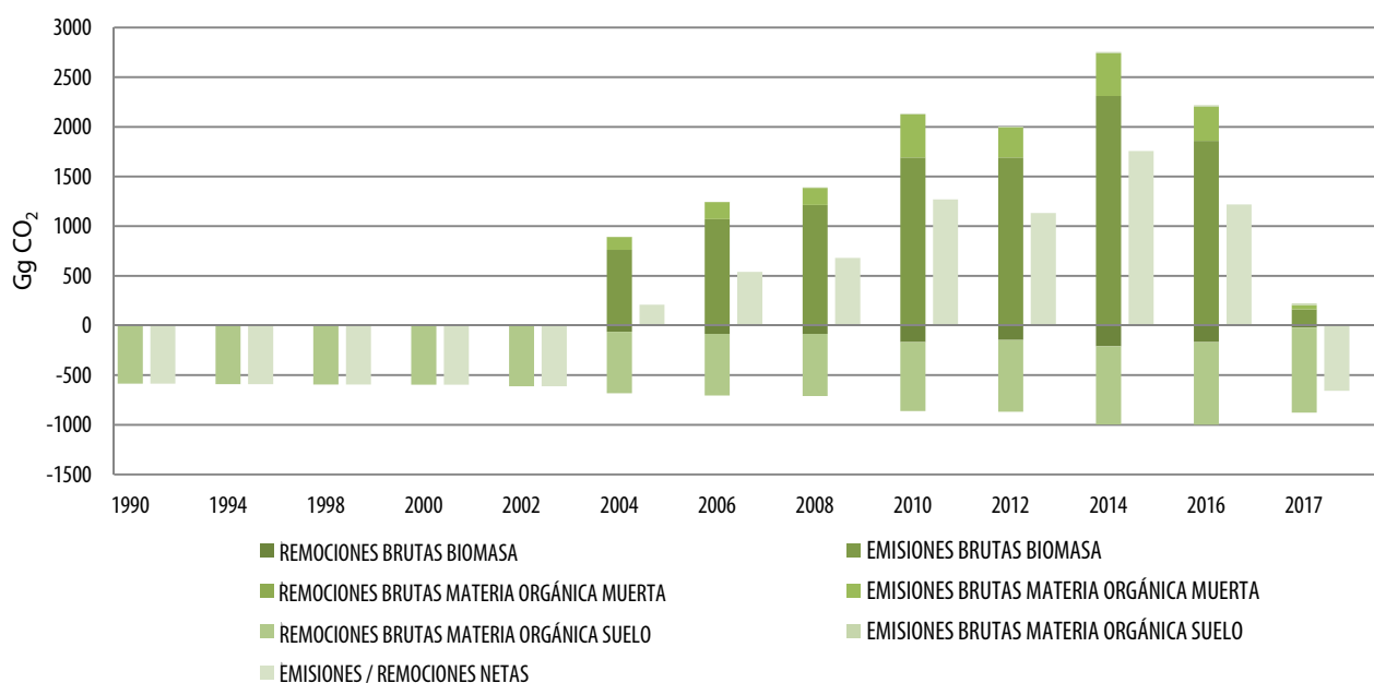
Figura 18. Evolución de las emisiones brutas, remociones brutas y emisiones / remociones netas de CO 2 , por reservorio de carbono, en Tierras convertidas a Pastizales, período 1990-2017
