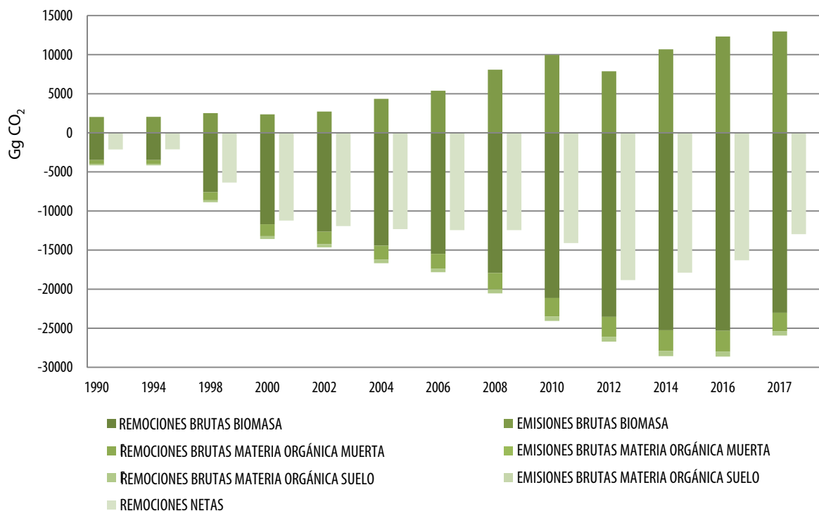
Figura 12. Evolución de las emisiones brutas, remociones brutas y remociones netas de CO 2 , por reservorio de carbono, en Tierras convertidas a Tierras forestales, período 1990-2017
