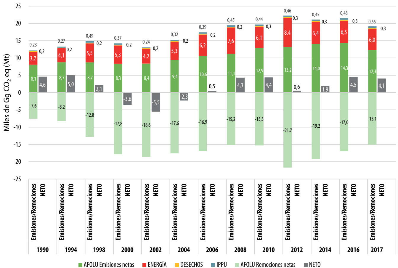
Figura 27. Evolución de emisiones, por sector. Métrica GTP 100 AR5
