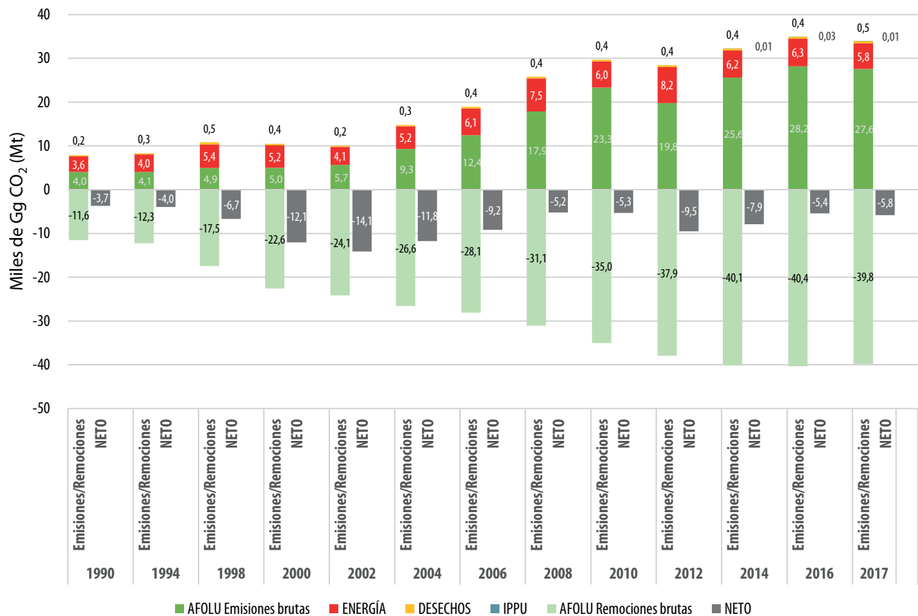
Figura 25. Evolución de emisiones de CO 2 por sector, 1990-2017
