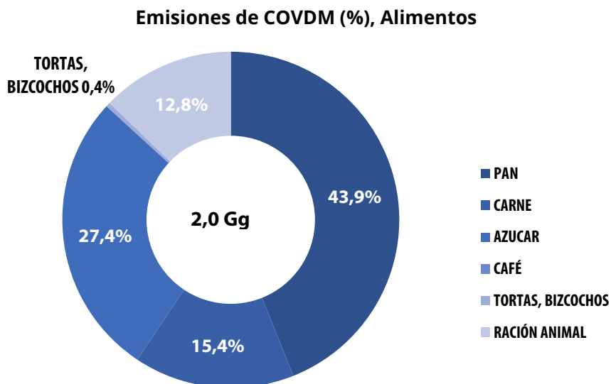
Figura 25. Emisiones de COVDM (%), Alimentos del sector IPPU
