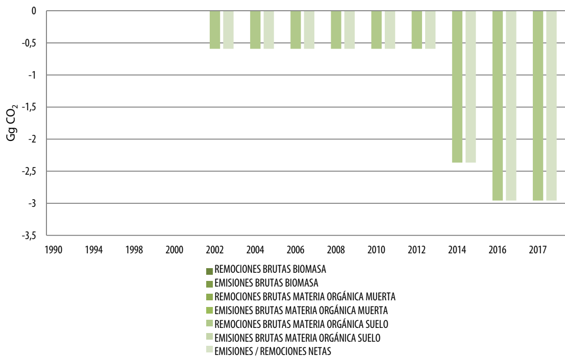
Figura 22. Evolución de las emisiones brutas, remociones brutas y emisiones / remociones netas de CO 2 , por reservorio de carbono, en Tierras convertidas a Otras tierras, período 1990-2017
