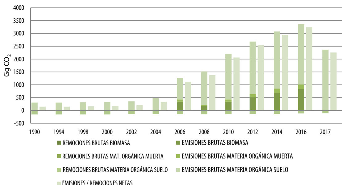
Figura 15. Evolución de las emisiones brutas, remociones brutas y emisiones / remociones netas de CO 2 , por reservorio de carbono, en Tierras convertidas a Tierras de cultivo, período 1990-2017
