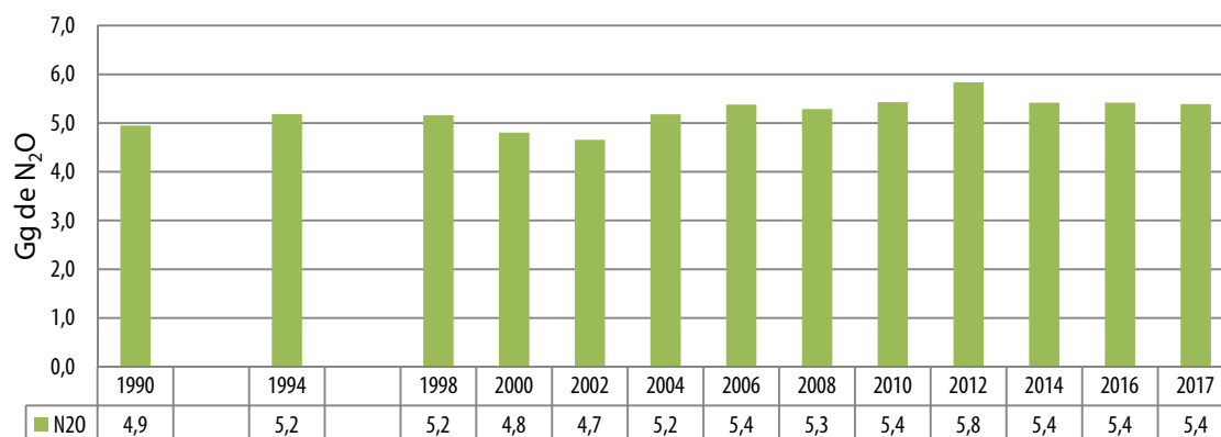
Figura 28. Evolución de las Emisiones indirectas de óxido nitroso en suelos agropecuarios para el período 1990-2017.
