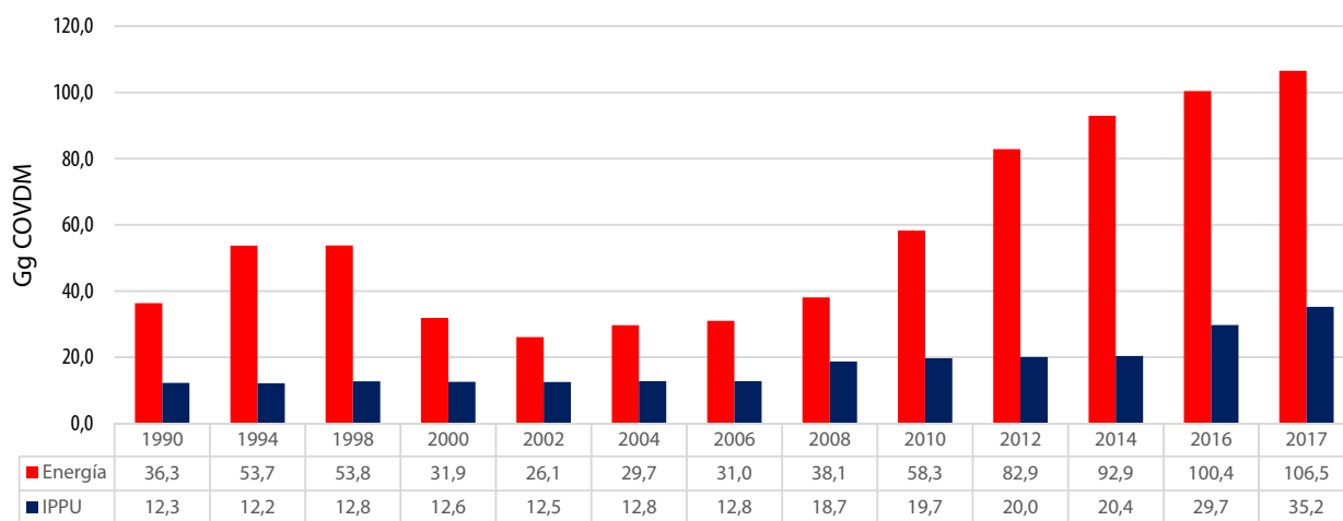
Figura 7. Evolución de emisiones nacionales de COVDM, 1990-2017.
