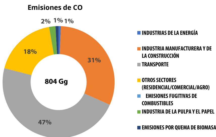
Figura 2. Emisiones nacionales de CO por categoría, 2017
