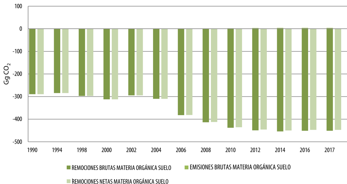
Figura 17. Evolución de las emisiones brutas, remociones y remociones netas de CO 2 de Pastizales que permanecen como Pastizales, período 1990-2017
