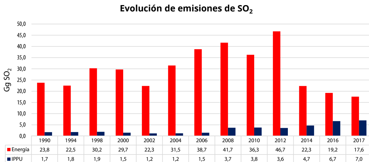
Figura 8. Evolución de emisiones nacionales de SO 2 , 1990-2017
