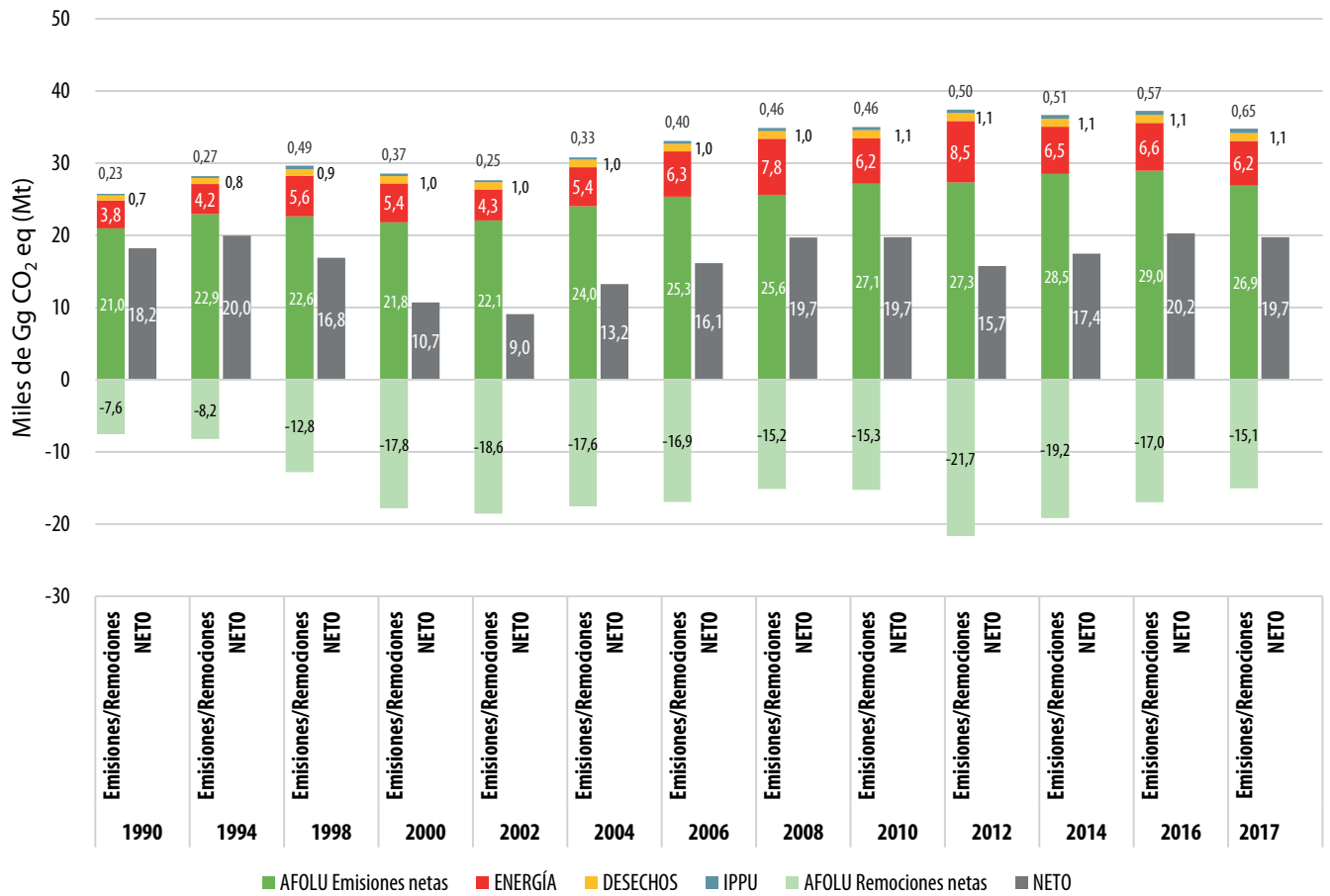
Figura 26. Evolución de emisiones, por sector. Métrica GWP 100 AR2
