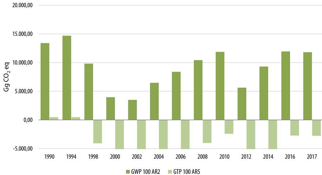
Figura 4. Evolución de emisiones del Sector AFOLU, en Gg de CO 2 eq considerando las métricas GWP 100 AR2 y GTP 100 AR5 , para el período 1990-2017
