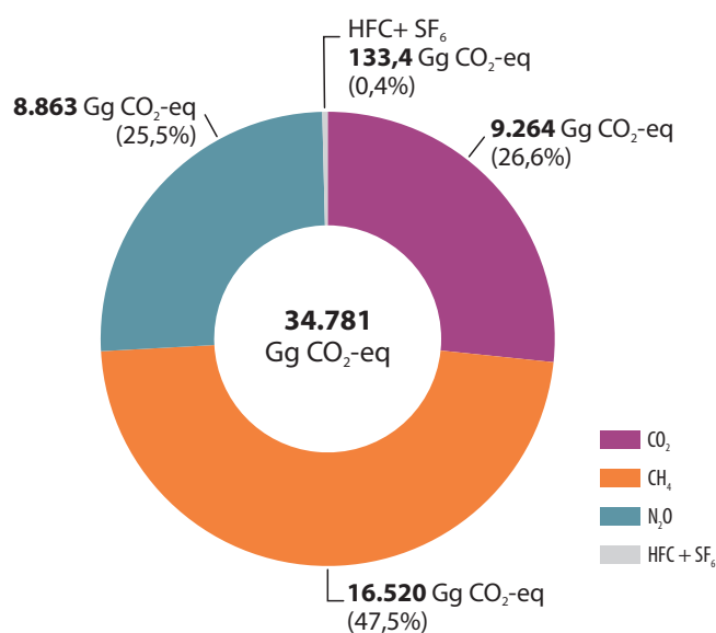
Figura 8. Contribución de emisiones por gas (sin considerar aportes de categorías con remociones netas), 2017, GWP 100 AR2
