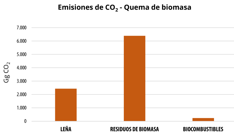
Figura 21: Emisiones de CO 2 de Quema de biomasa por energético, 2017.
