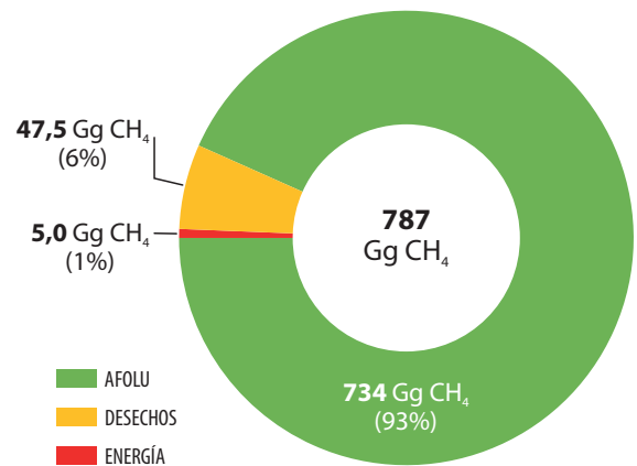
Figura 6. Emisiones nacionales de CH 4 por sector, 2017
