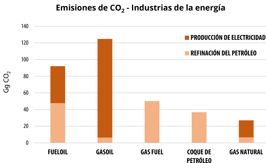
Figura 14: Emisiones de CO 2 de Industrias de la energía por combustible, 2017.
