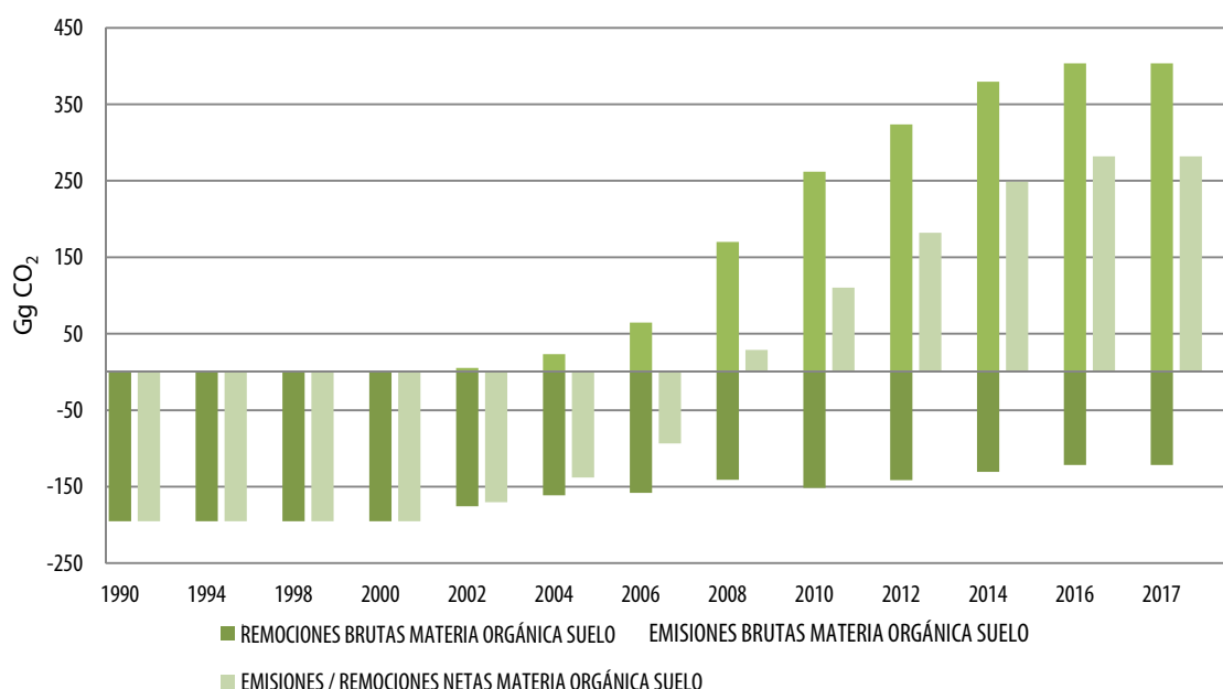
Figura 14. Evolución de emisiones brutas, remociones brutas y emisiones / remociones netas en Tierras de cultivo que permanecen como Tierras de cultivo, período 1990-2017
