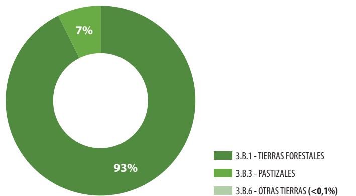
Figura 20. Contribución relativa de remociones de CO 2 , del sector AFOLU, 2017.
