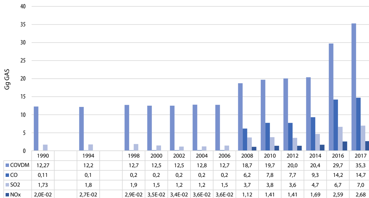
Figura 7. Evolución de emisiones GEI indirectos, sector IPPU
