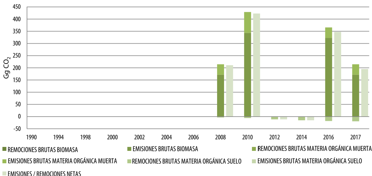
Figura 20. Evolución de las emisiones brutas, remociones brutas y emisiones / remociones netas de CO 2 , por reservorio de carbono, en Tierras convertidas a Asentamientos, período 1990-2017
