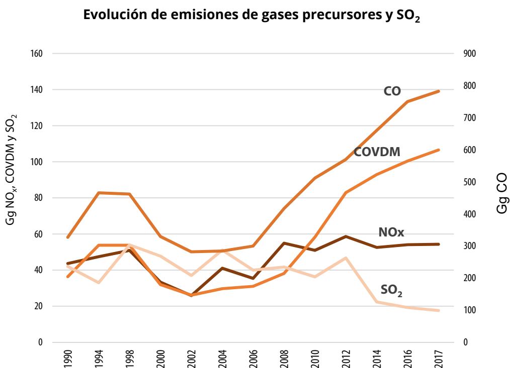
Figura 27: Evolución de las emisiones de gases precursores (IPCC 1996 rev.) y SO 2 , período 1990-2017.
