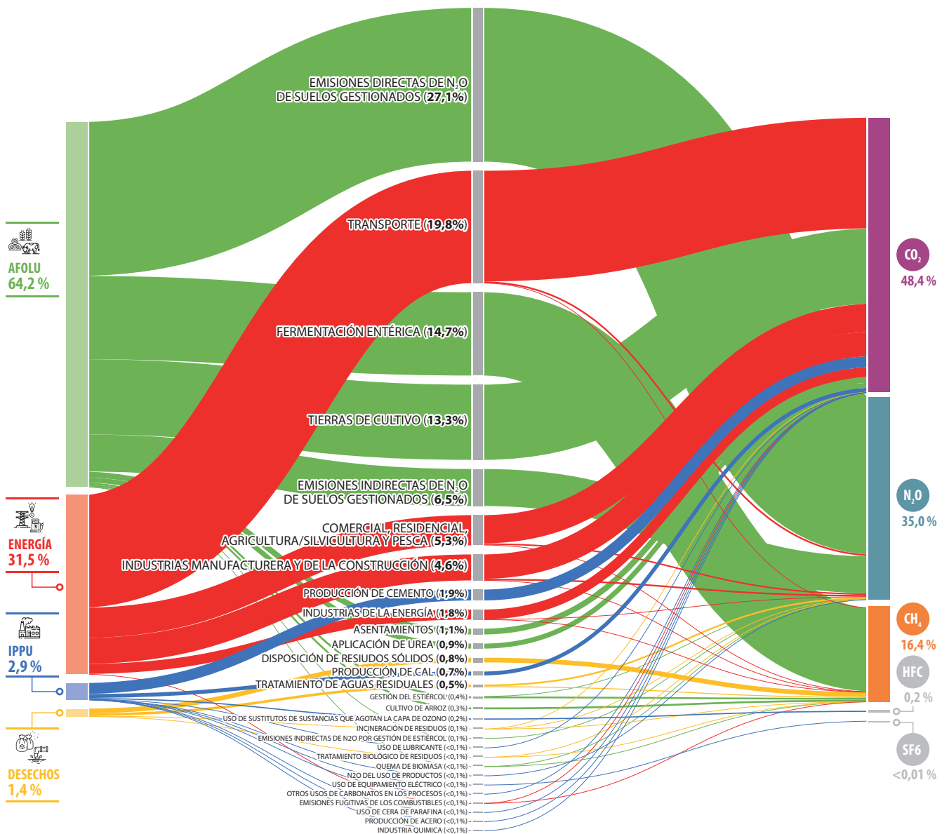
Figura 11. Distribución de emisiones nacionales por sector y categoría con métrica GTP_{100\text{ AR5}} 2017
