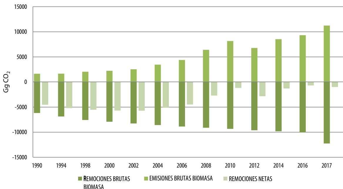
Figura 11. Emisiones brutas, remociones brutas y remociones netas de CO 2 en Tierras forestales que permanecen como Tierras forestales, período 1990-2017
