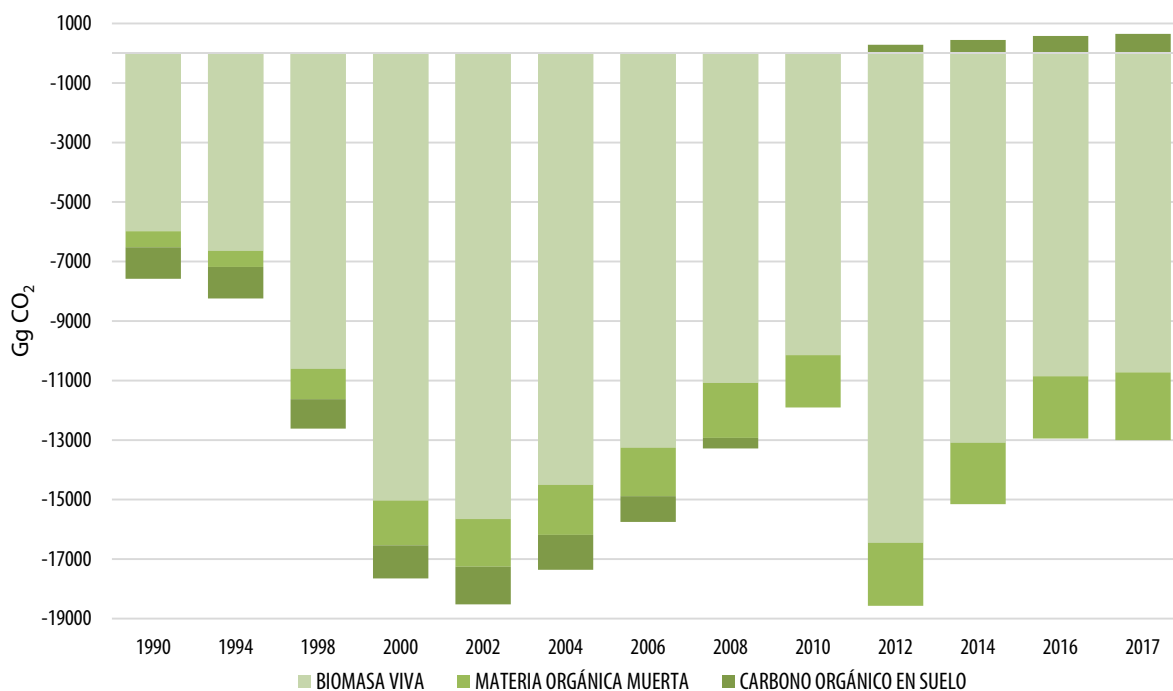
Figura 9. Evolución de las emisiones / remociones netas de CO 2 por reservorio de carbono para la serie temporal 1990-2017
