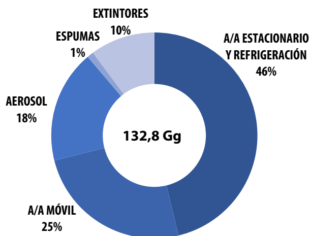
Figura 20. Distribución de emisiones de HFC por aplicación en CO_2 -eq del sector IPPU, métrica GWP_{100, AR2}
