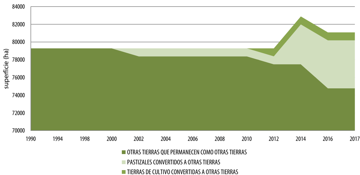
Figura 21. Evolución de la superficie ocupada por Otras tierras, discriminado por subcategoría, período 1990-2017
