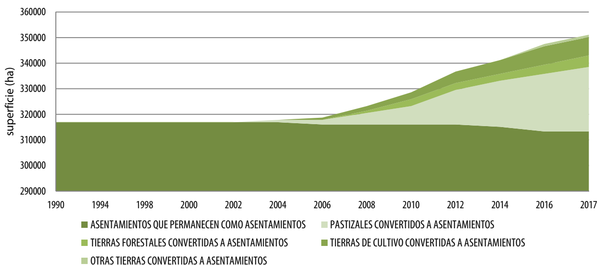
Figura 19. Evolución de la superficie ocupada por Asentamientos, discriminado por subcategoría, período 1990-2017
