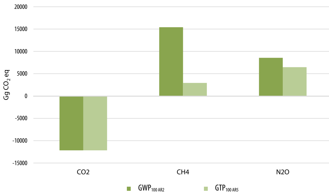
Figura 2. Emisiones / remociones netas por gas del sector AFOLU, 2017
