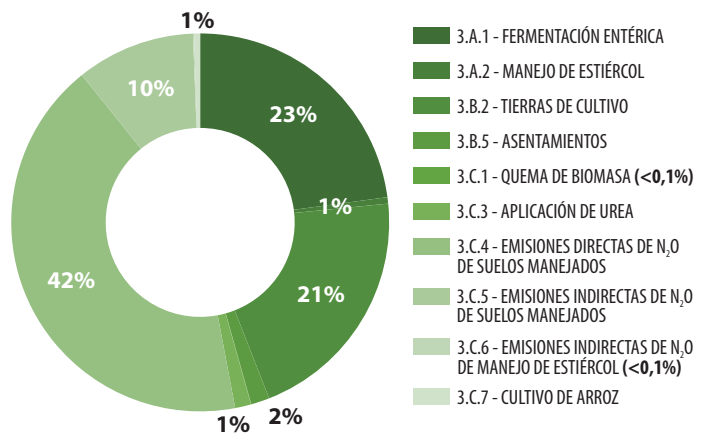
Figura 19. Contribución relativa de emisiones GEI, del sector AFOLU, por categoría, 2017 (GTP 100 AR5 )
