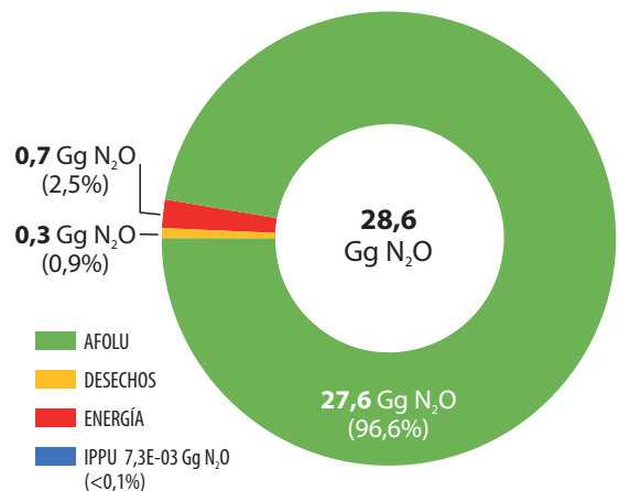
Figura 7. Emisiones nacionales de N 2 O por sector, 2017
