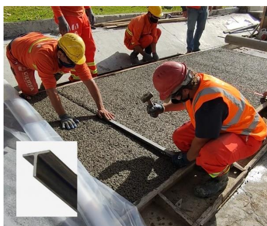
Figura 29. Instalación de juntas mediante perfil tee.
