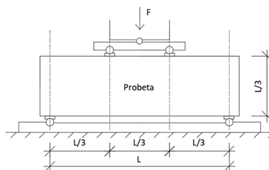
Figura 13. Esquema del ensayo de flexión a cuatro puntos.
