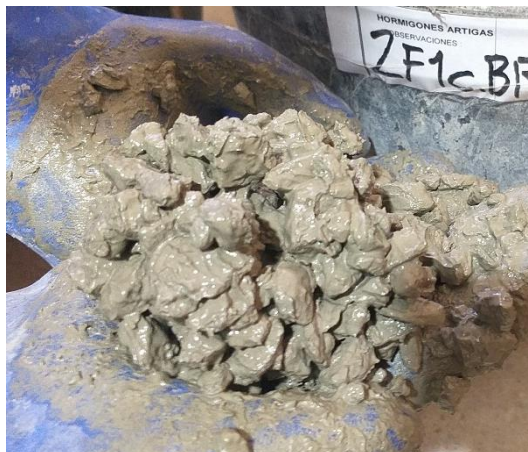
Figura 18. Mezcla de hormigón permeable con cantidad excesiva de agua.
