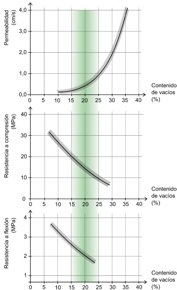
Figura 9. Valores típicos de permeabilidad, resistencia a compresión y resistencia a flexión en función del contenido de vacíos para el hormigón permeable.
