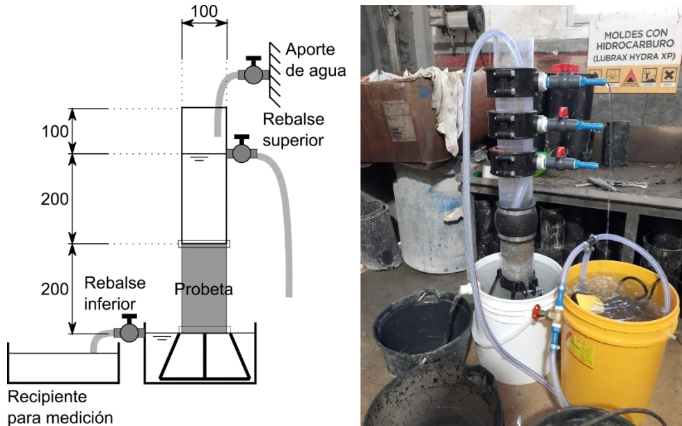
Figura 11. Esquema e imagen del permeámetro de carga constante.
