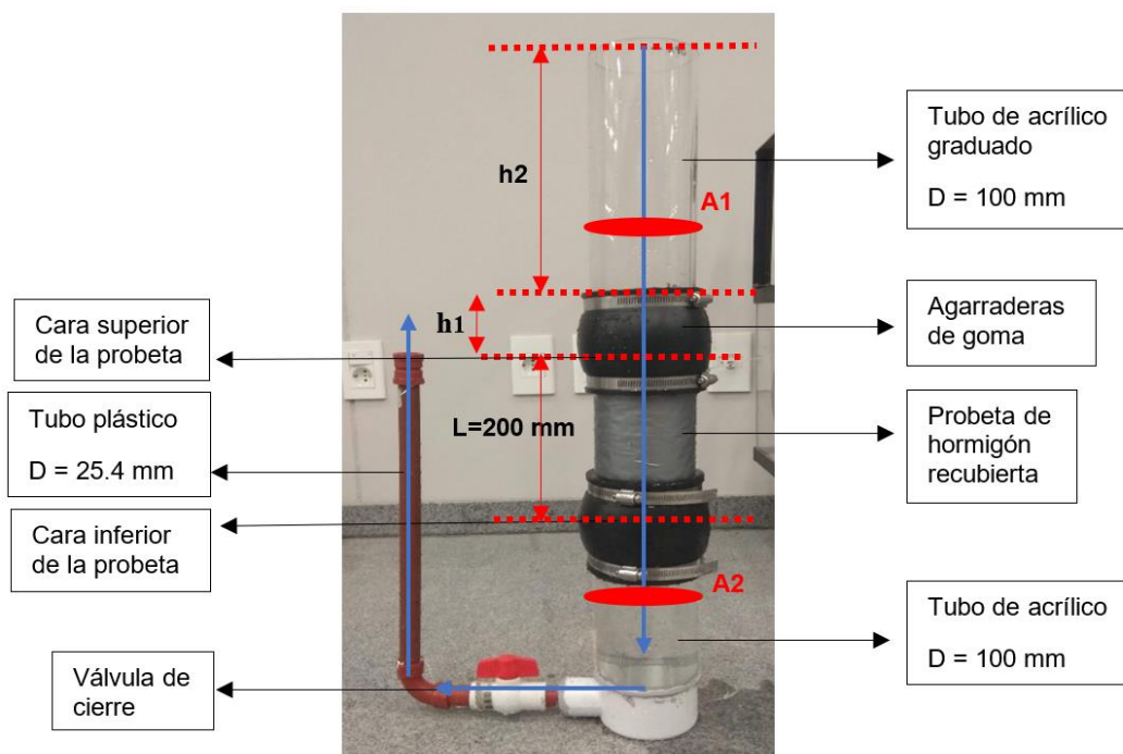
Figura 10. permeámetro de carga variable.
