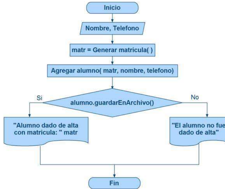
Figura 11-7: Diagrama de flujo del algoritmo para dar de alta a un alumno
