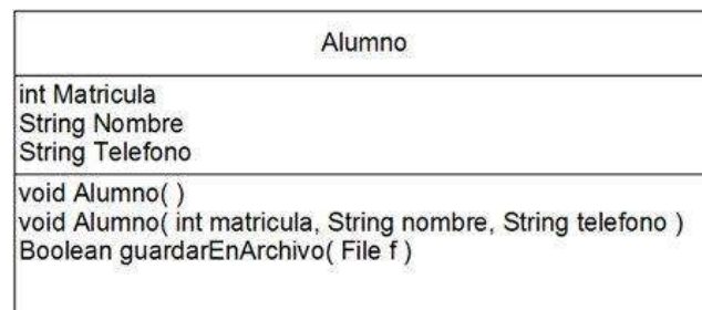
Figura 11-6: La clase Alumno
