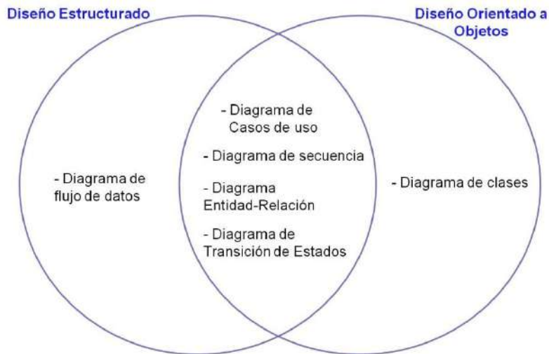
Figura 5-9: Modelos para el Diseño Estructurado y el Diseño Orientado a Objetos
