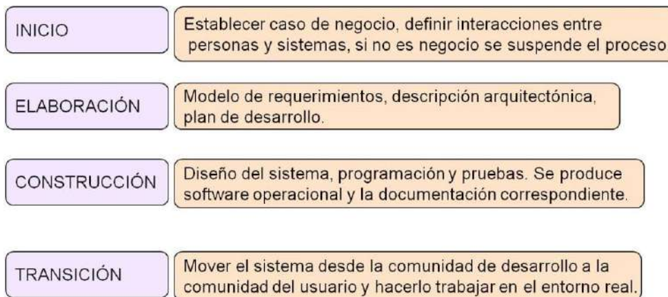
Figura 12-4: Descripción de las Fases del Proceso Unificado
