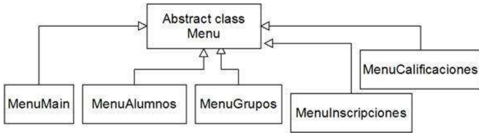
Figura 11-4: Diagrama de clases de los menús del sistema
