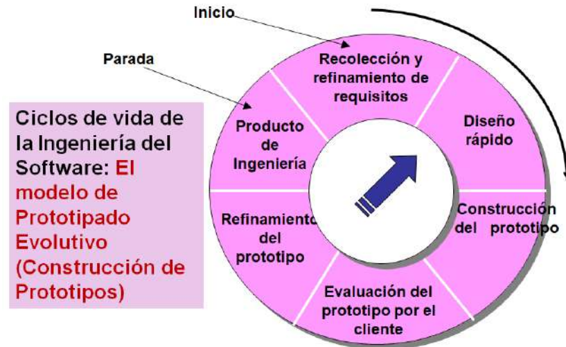
Figura 10-4: El prototipado evolutivo
