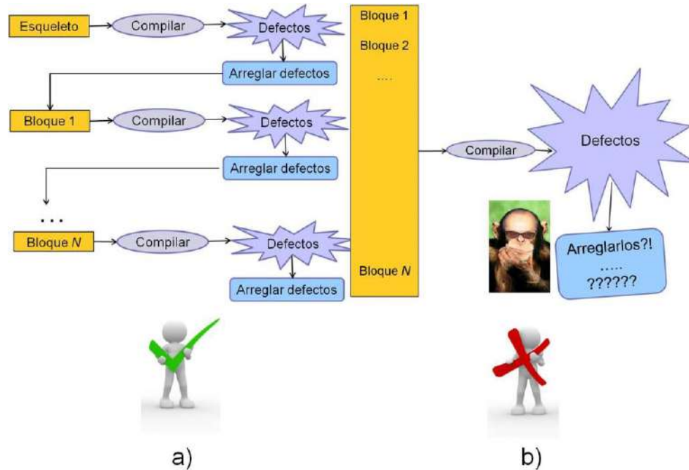
Figura 6-2: Buena y mala práctica de codificación-compilación
