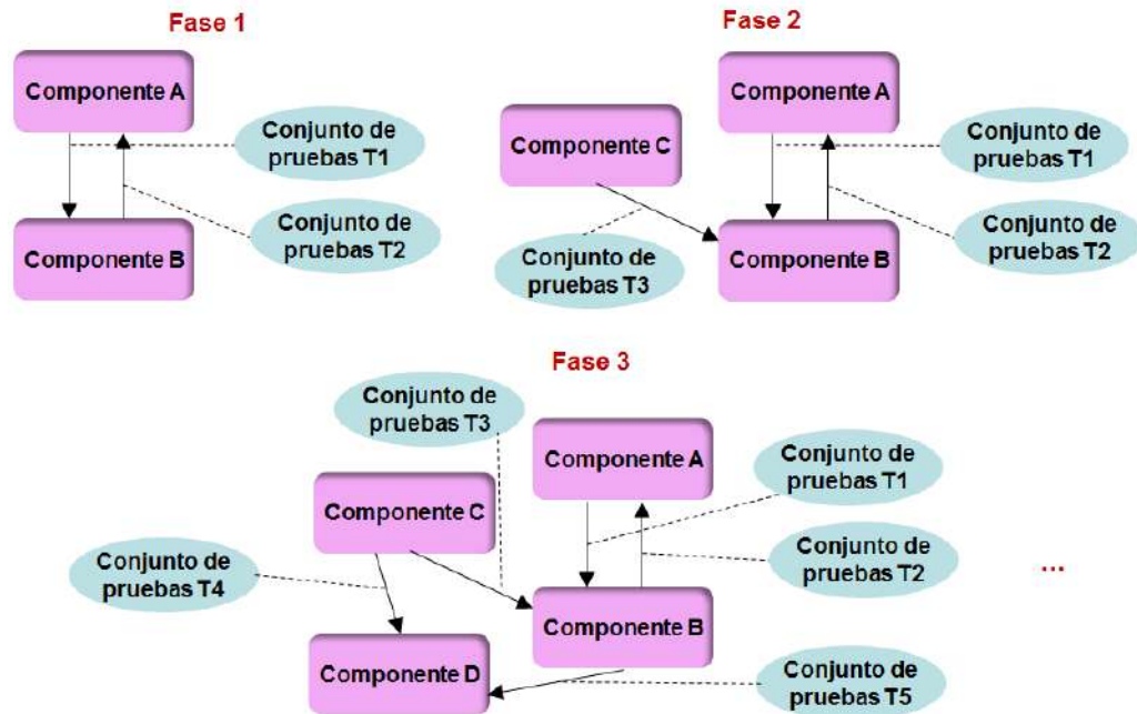
Figura 8-5: Proceso incremental de pruebas de integración
