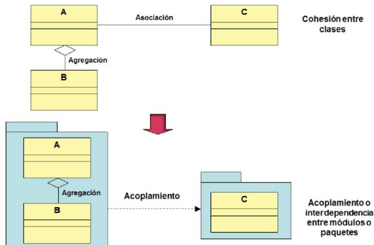
Figura 5-16: Ejemplo de cohesión y acoplamiento entre clases
