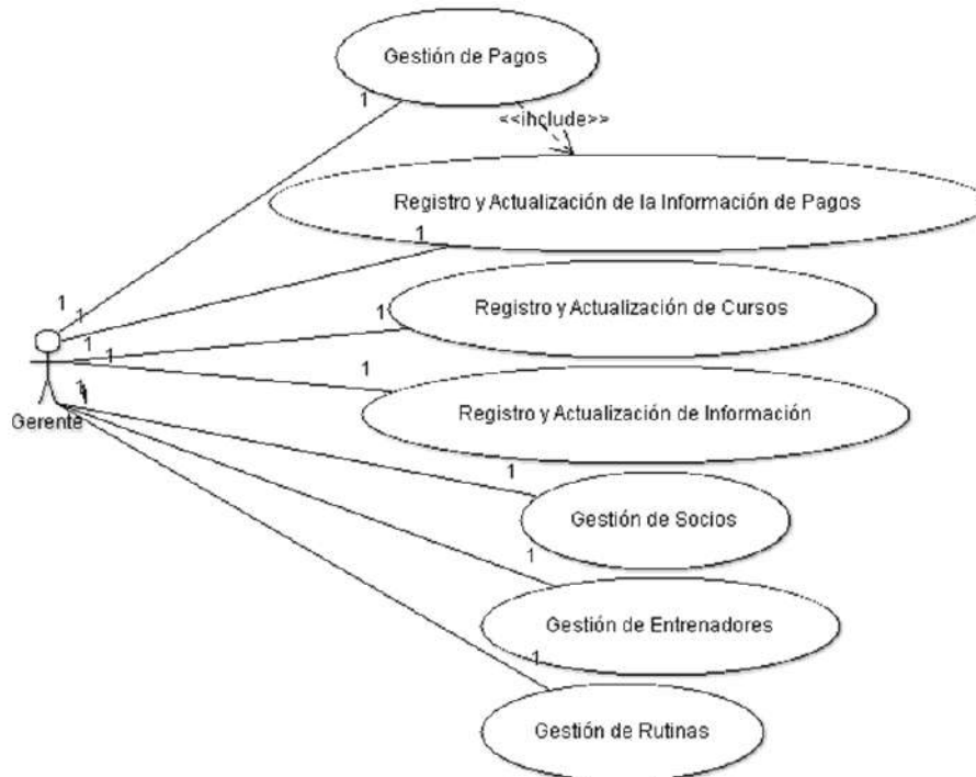
Figura 5-26: Ejemplo de artefacto (diagrama de casos de uso)
