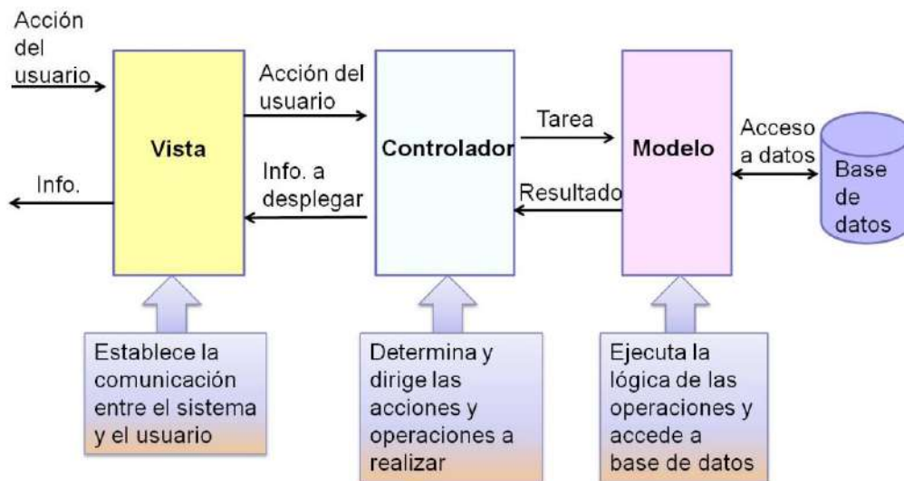
Figura 5-18: Modelo-Vista-Controlador (MVC)
