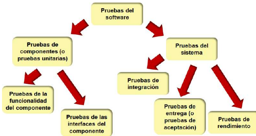
Figura 8-4: Algunos tipos de pruebas del software
