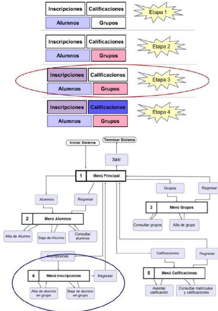
Figura 11-21: En la tercera etapa se desarrolla funcionalidad para el Menú Inscripciones
