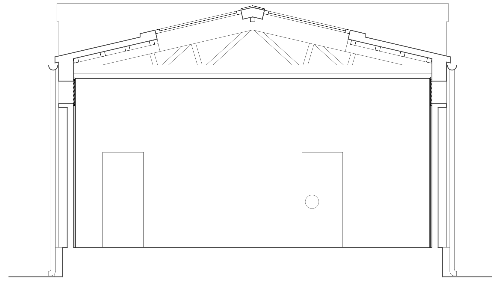
SEZIONE C-C
