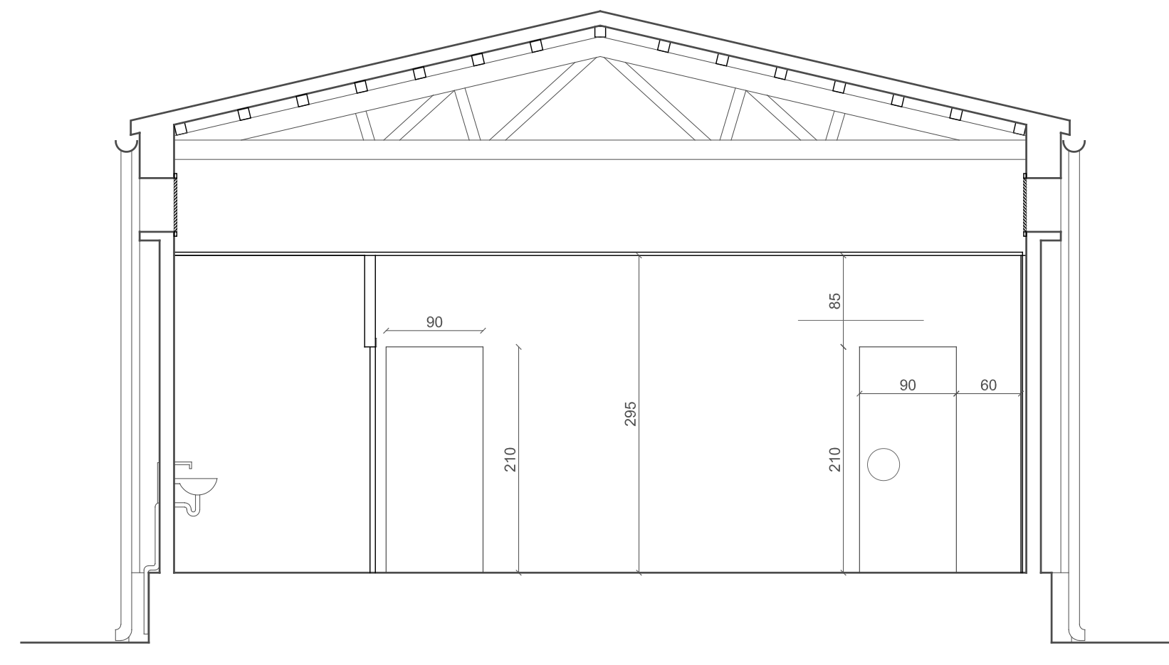
SEZIONE B-B
