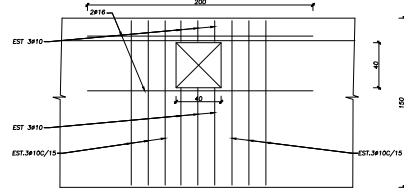
DETALLE PASE EN VIGAS DE FACHADA EN BLOQUE ASUNCIÓN ESC. 1 : 20
