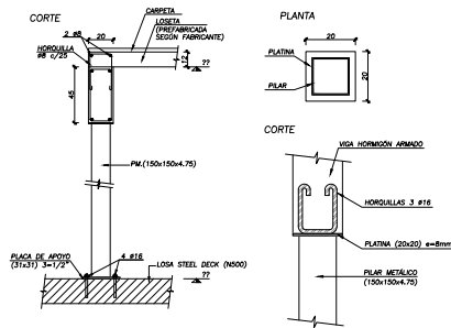
PILARES METÁLICOS N600 BLOQUE ASUNCIÓN ESC. 1 : 20
