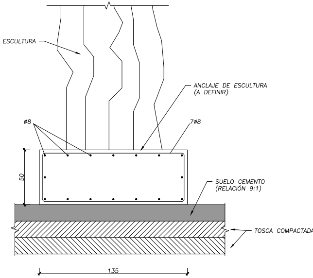
DETALLE BASE ESCULTURA ESC. 1 / 10
