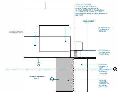
DETALLE ENCUENTRO MURO - PILAR 1 : 10
