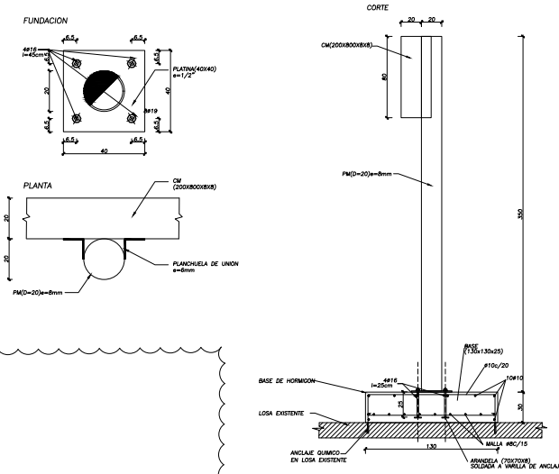
DETALLE BASE ESCULTURA ESC. 1 / 10
