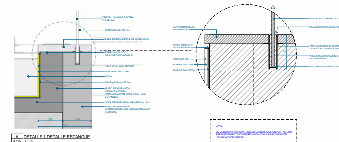
6 DETALLE 1 DETALLE ESTANQUE A715 1 : 10
