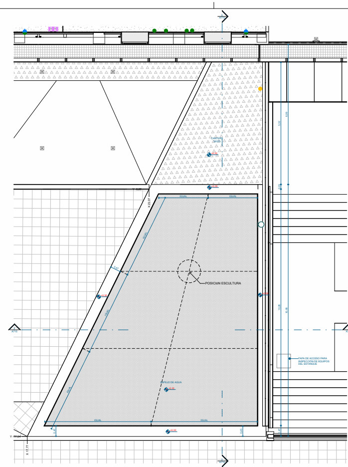
1 PLANTA DETALLE ESTANQUE A715 1 : 50
