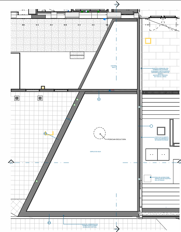
PLANTA DETALLE ESTANQUE MUROS 1:50
