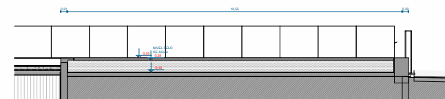
3 CORTE B DETALLE ESTANQUE A715 1 : 50
