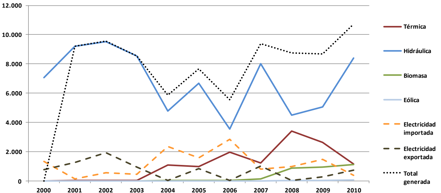
Generación de energía eléctrica conectada al S.I.N. (GWh)
