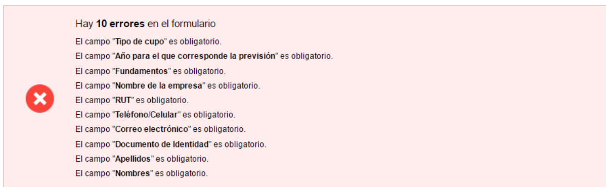
Figura 12. Errores detectados.
