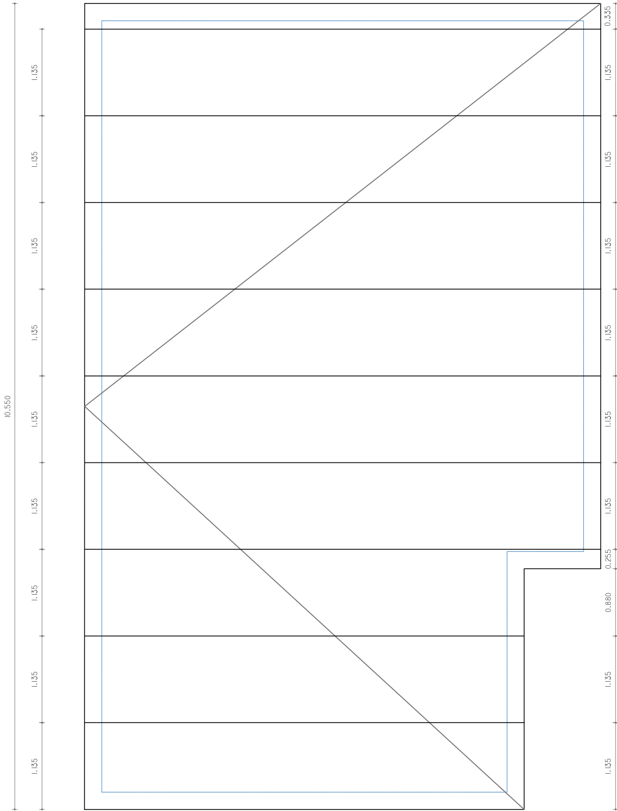
PLANTA DE TECHOS ESCALA_1/50
