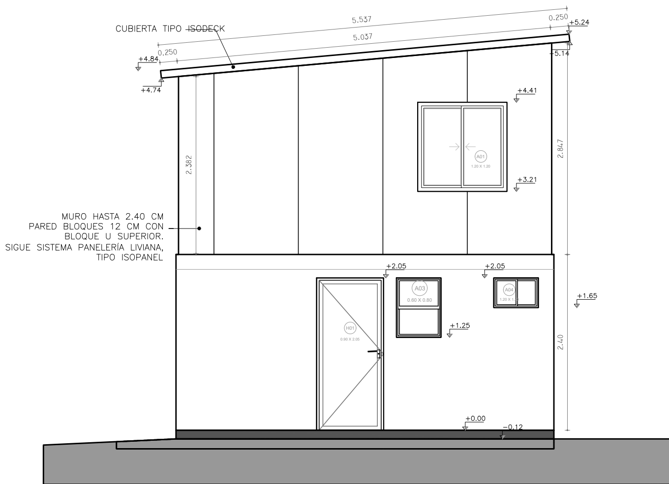
FACHADA FONDO ESCALA_1/50
