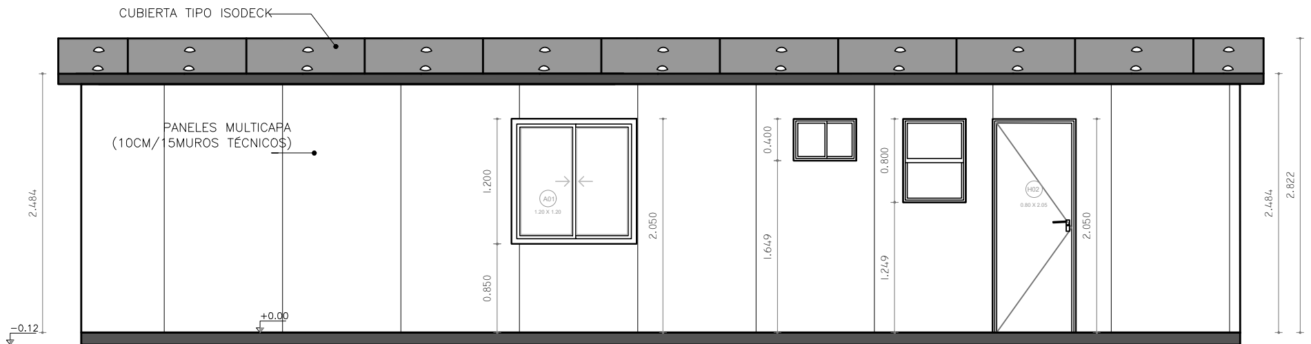
FACHADA FONDO ESCALA_1/50
