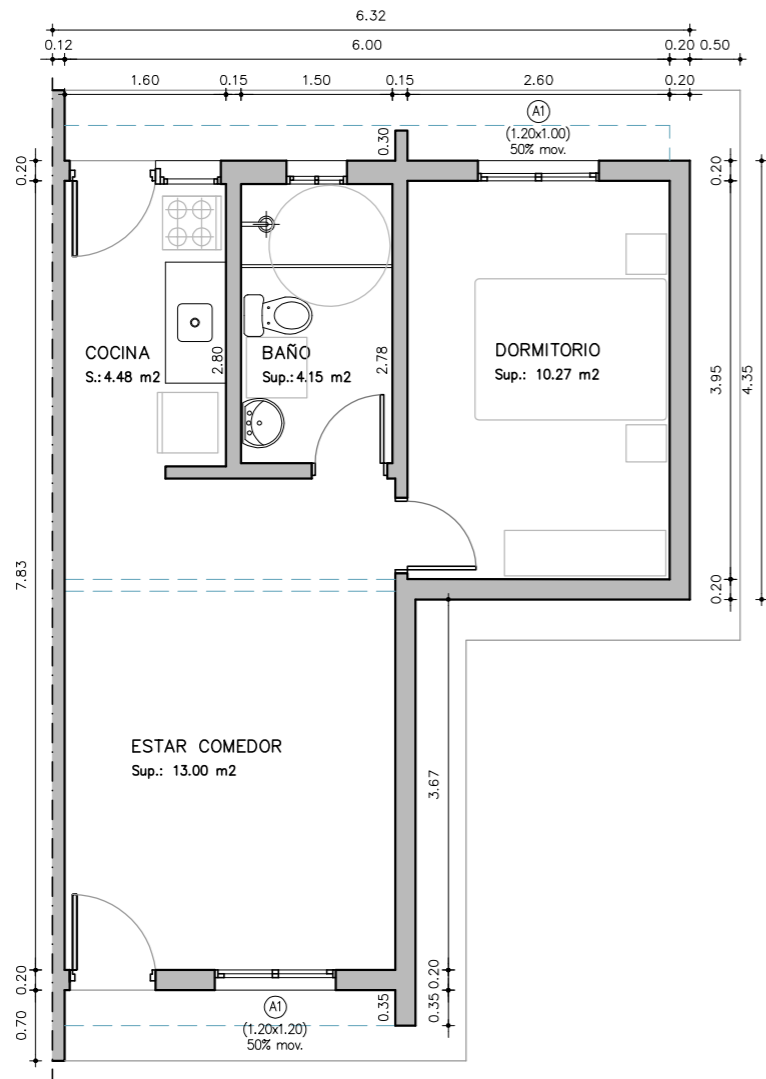
PLANTA TIPOLOGIA_1D ESCALA_1/75 SUP.: 41 m 2
