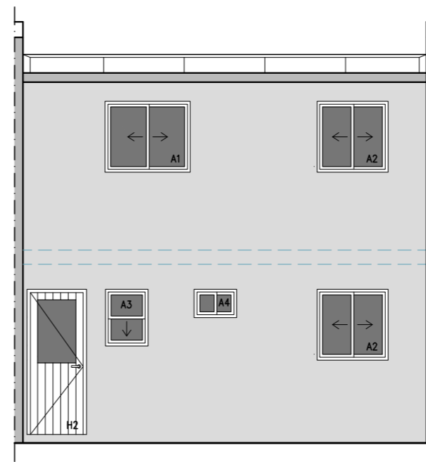
FACHADA_POSTERIOR ESCALA_1/75 SUP.: 88 m2
