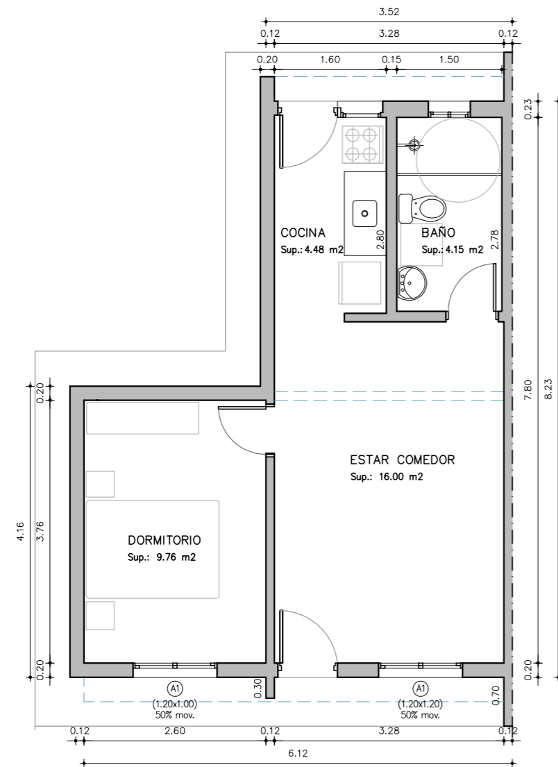
PLANTA_TIPOLOGIA_1D ESCALA_1/50 SUP.: 41 m 2
