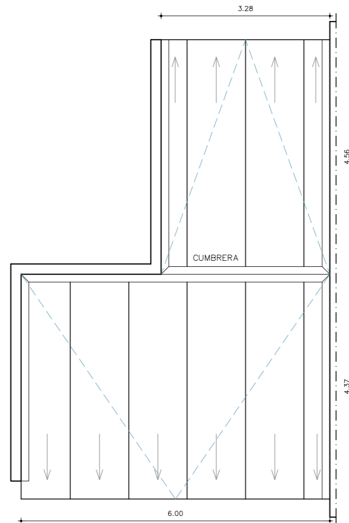
PLANTA_TECHOS_1D ESCALA_1/75 SUP.: 41 m 2
