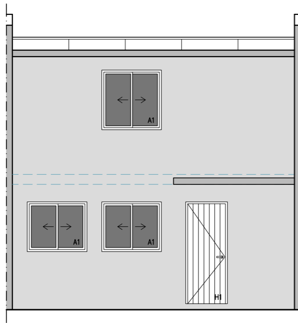
FACHADA_PRINCIPAL ESCALA_1/75 SUP.: 80 m2
