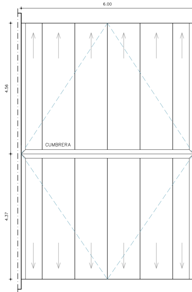
PLANTA TECHOS_2D ESCALA_1/75 SUP.: 51 m 2
