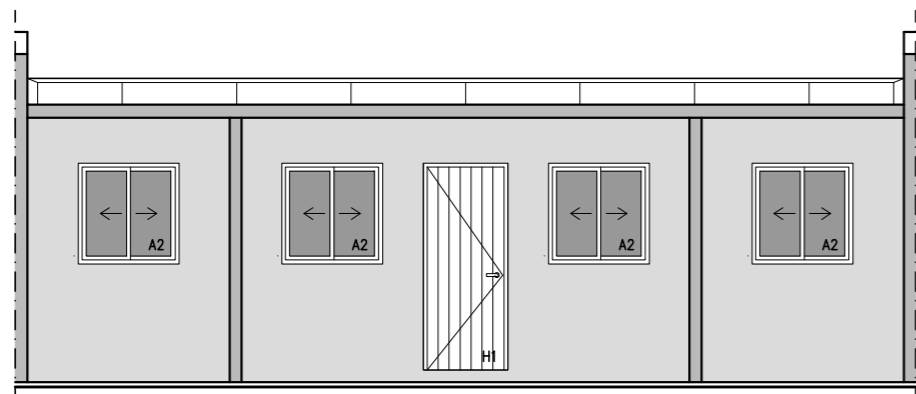
FACHADA_PRINCIPAL ESCALA_1/75 SUP.: 73 m2
