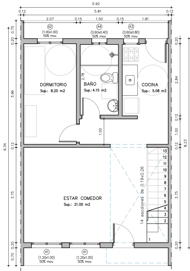
PLANTA_BAJA_TIPOLOGIA_3D_DUPLEX ESCALA_1/75 SUP.80 m2
