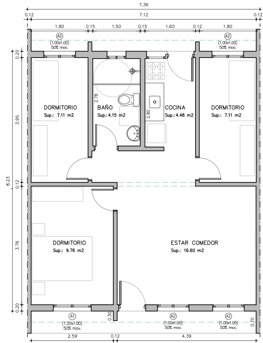
PLANTA TIPOLOGIA_3D ESCALA_1/75 SUP.: 60 m2
