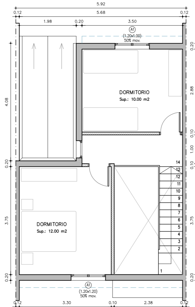
PLANTA_ALTA_TIPOLOGIA_3D_DUPLEX ESCALA_1/75 SUP.80 m2
