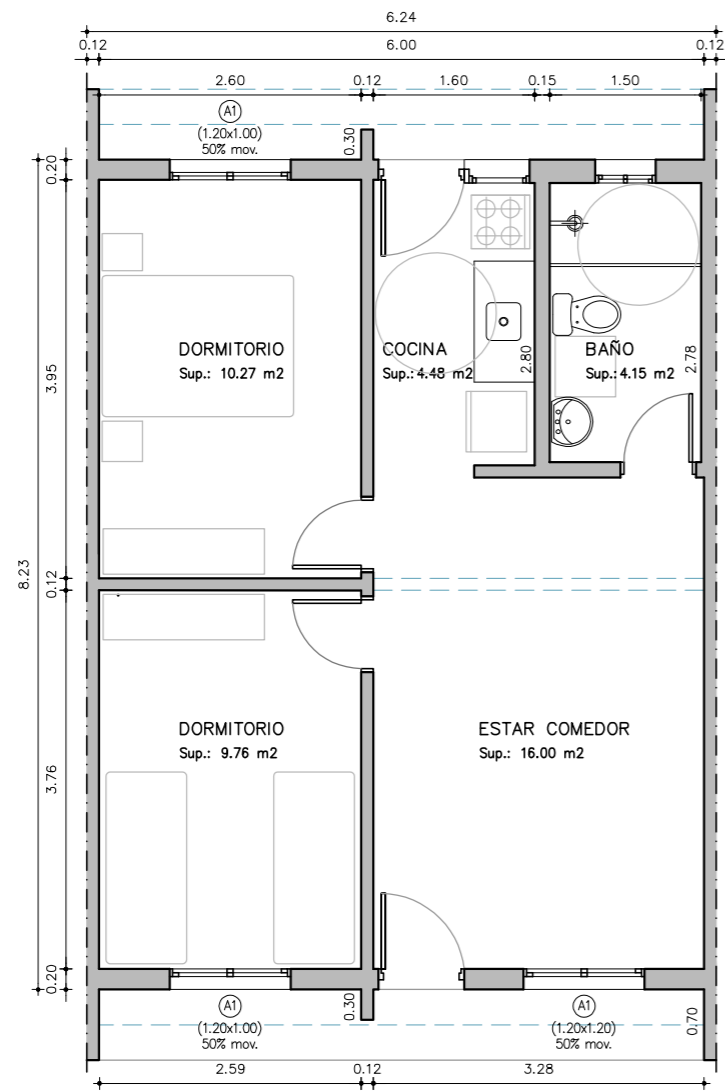
PLANTA TIPOLOGIA_2D ESCALA_1/75 SUP.: 51 m 2
