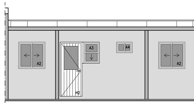
FACHADA POSTERIOR ESCALA_1/75 SUP.: 60 m2
