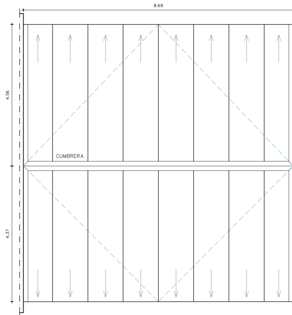
PLANTA_TECHOS_4D ESCALA_1/75 SUP.: 73 m2
