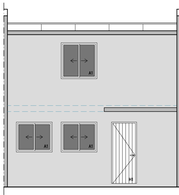
FACHADA_PRINCIPAL ESCALA_1/75 SUP.: 88 m2
