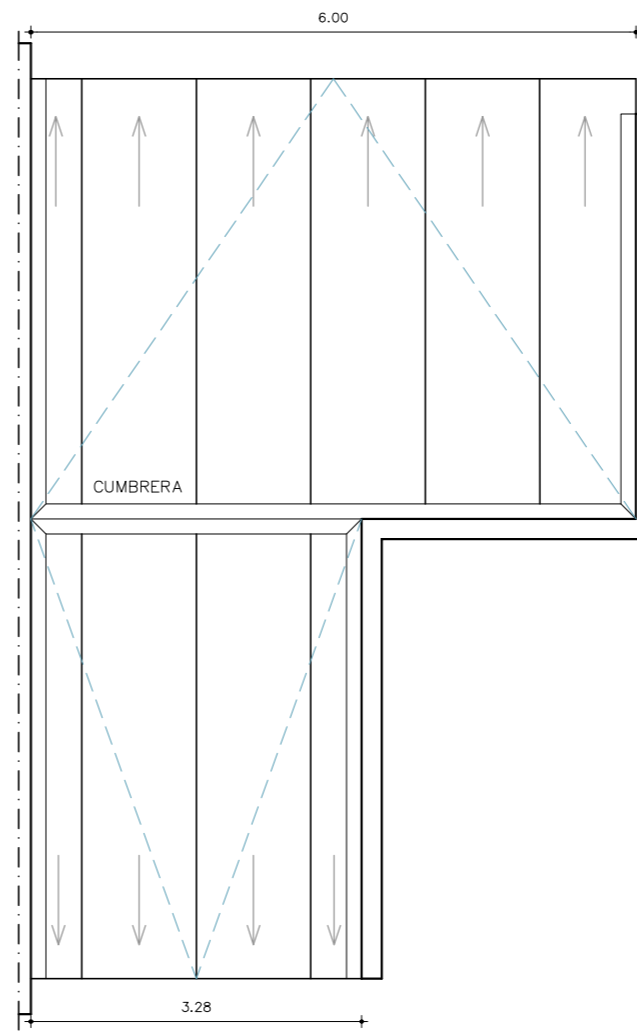
PLANTA TECHOS_1D ESCALA_1/75 SUP.: 41 m 2
