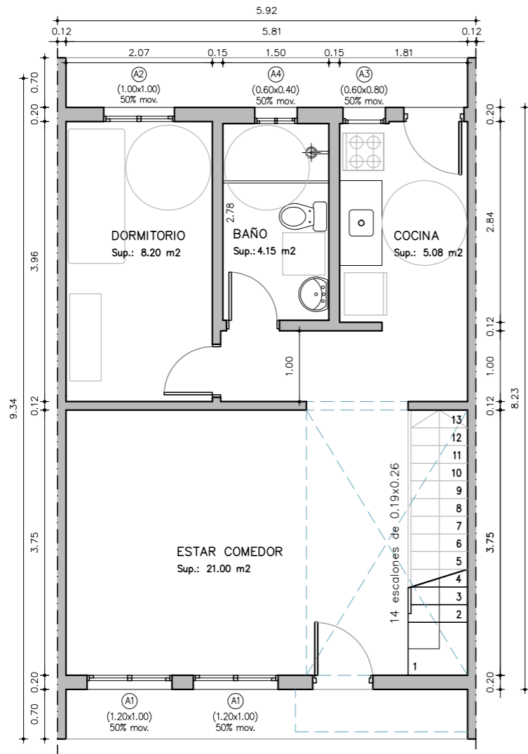
PLANTA_BAJA_TIPOLOGIA_4D_DUPLEX ESCALA_1/75 SUP.88 m2
