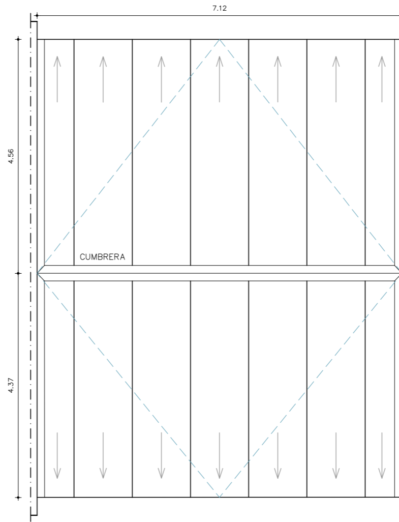
PLANTA TECHOS_3D ESCALA_1/75 SUP.: 60 m2
