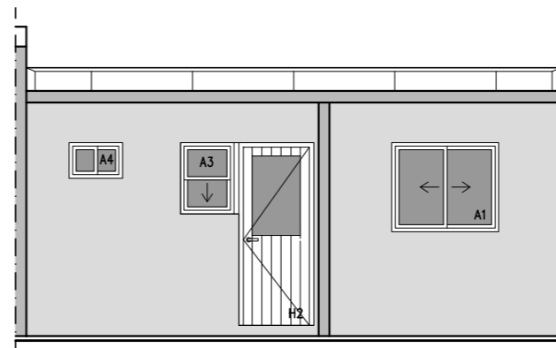
FACHADA POSTERIOR ESCALA_1/75 SUP.: 51 m 2
