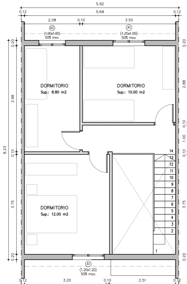
PLANTA_ALTA_TIPOLOGIA_4D_DUPLEX ESCALA_1/75 SUP.88 m2
