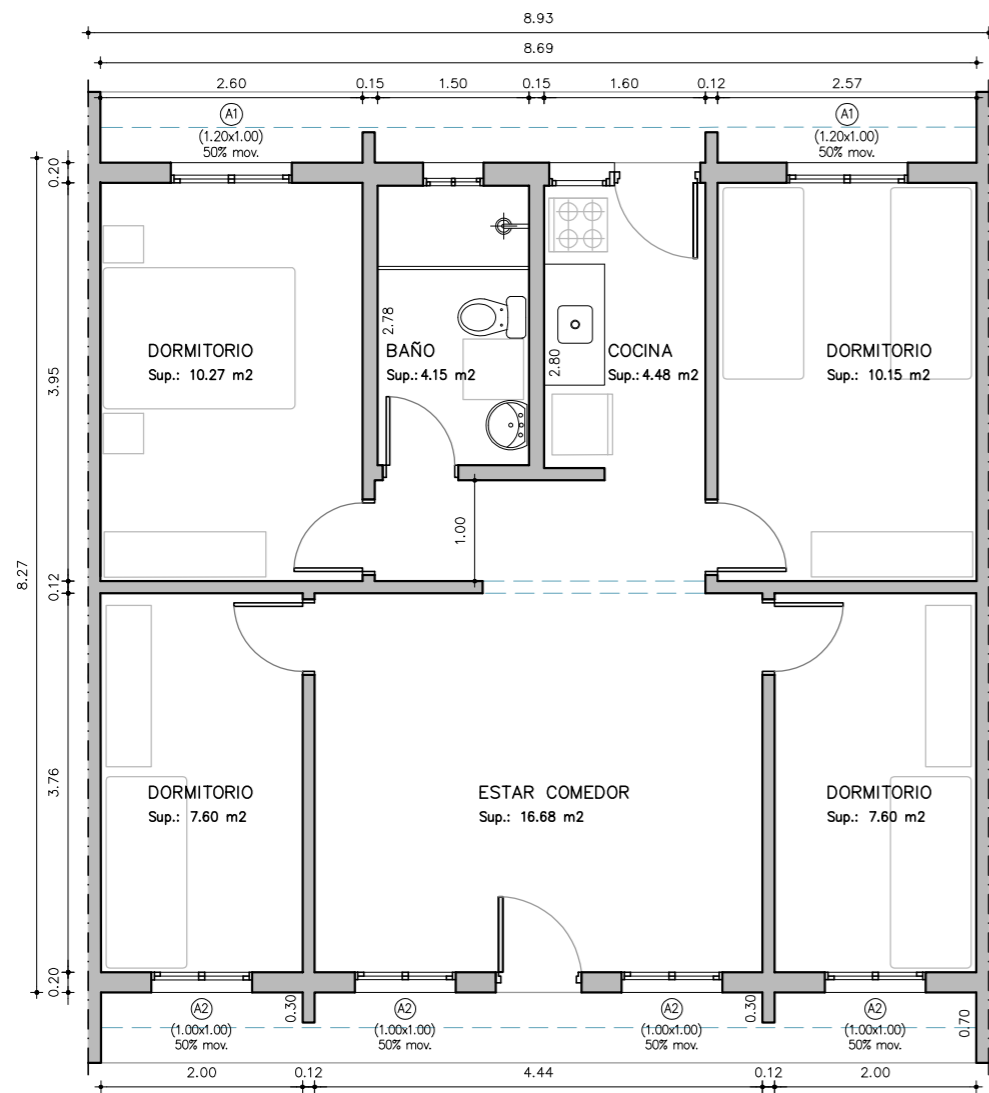
PLANTA_TIPOLOGIA_4D ESCALA_1/75 SUP.: 73 m2
