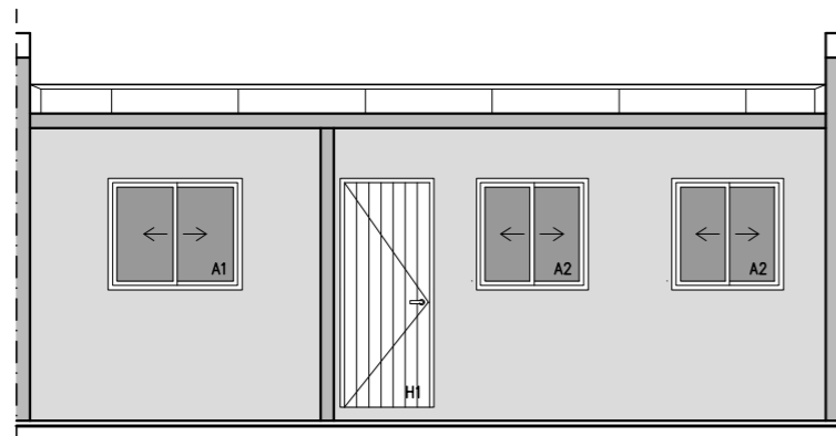
FACHADA PRINCIPAL ESCALA_1/75 SUP.: 60 m2
