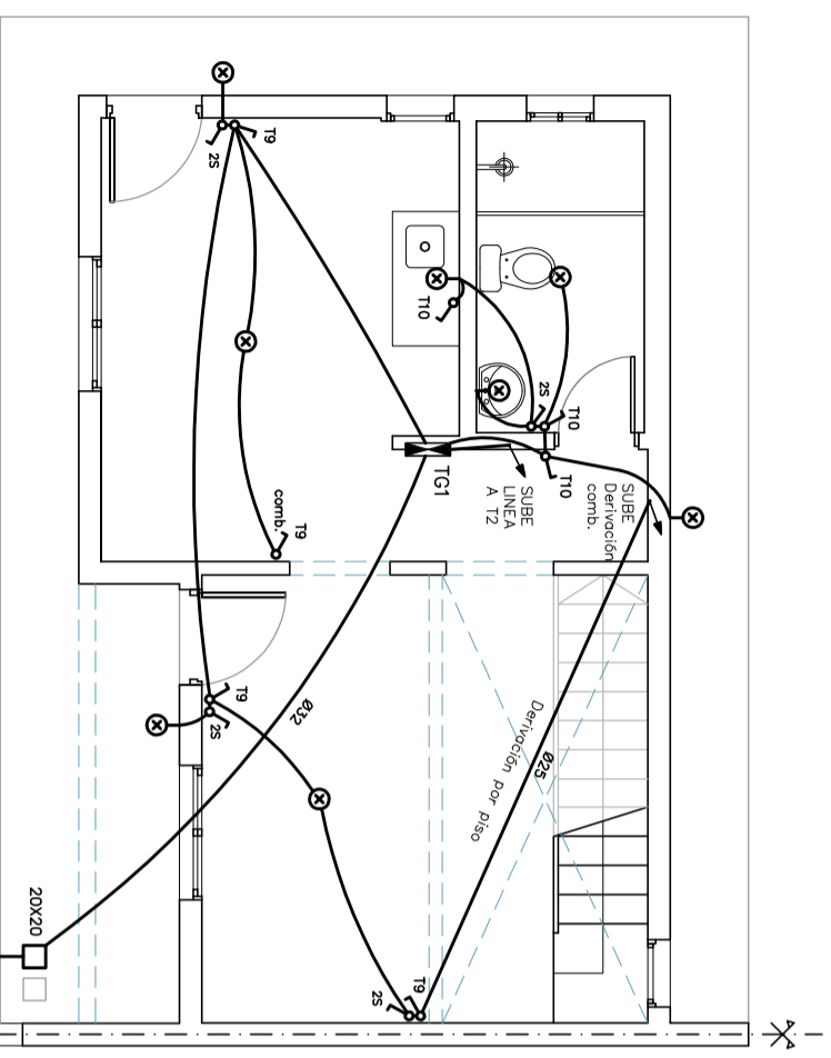
PLANTA_BAJA SISTEMA CONSTRUCTIVO TRADICIONAL
