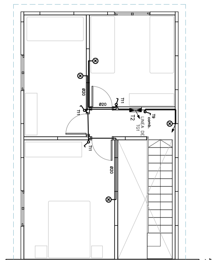
PLANTA_ALTA SISTEMA CONSTRUCTIVO PANELES MULTICAPA
