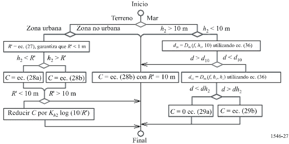
FIGURA 27 Organigrama para la corrección de altura de antena receptora/móvil
